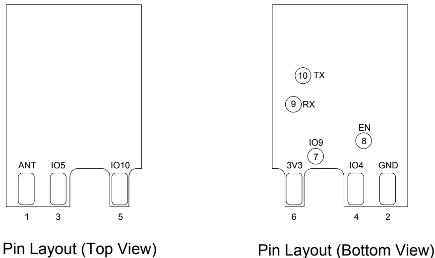
图 2: 管脚布局
