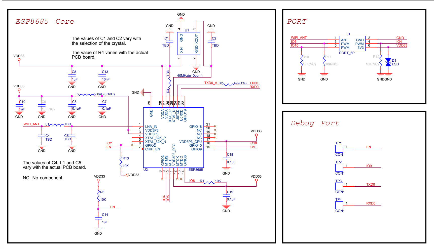
图 4: ESP8685-WROOM-07 原理图
