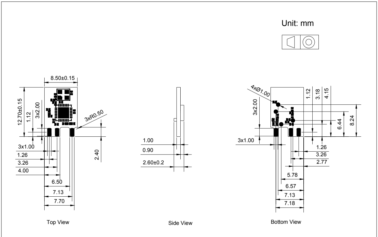
图 6: 模组尺寸
