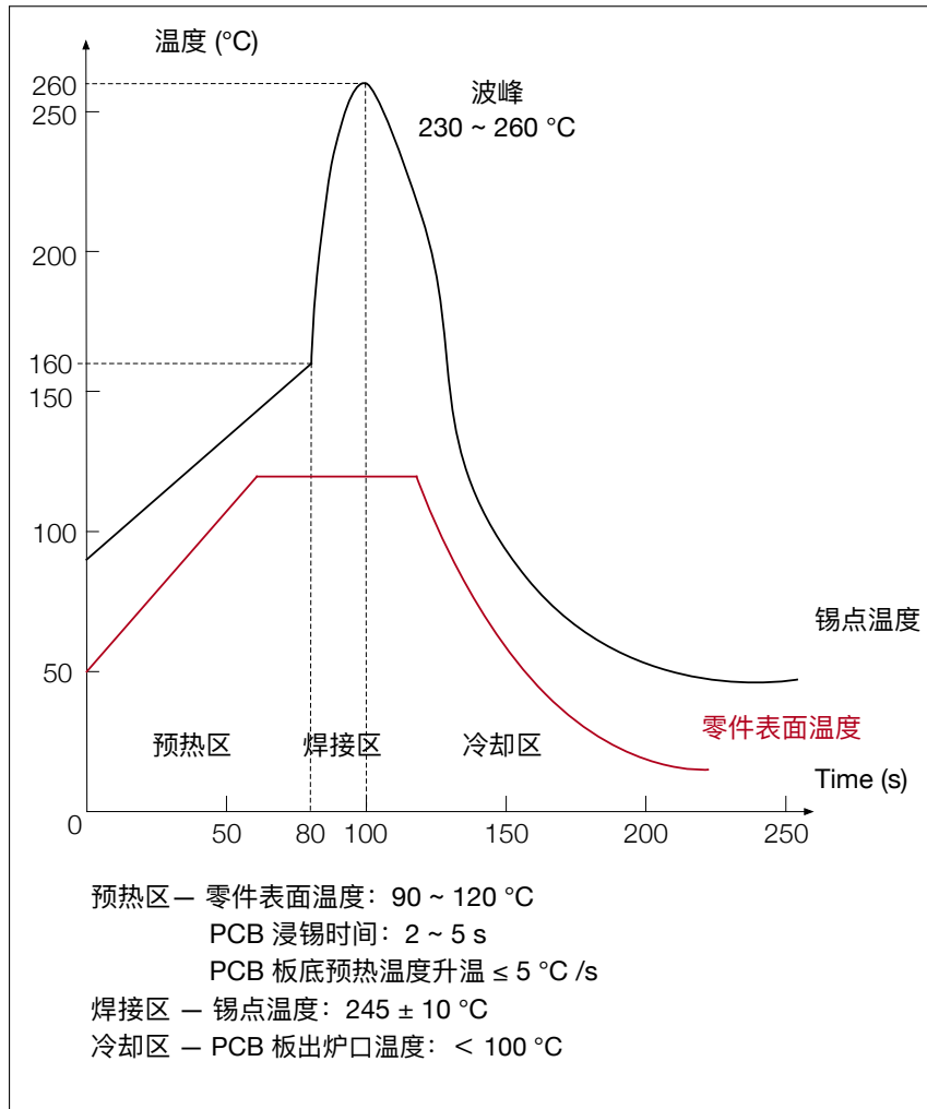
图 10: 波峰焊温度曲线
