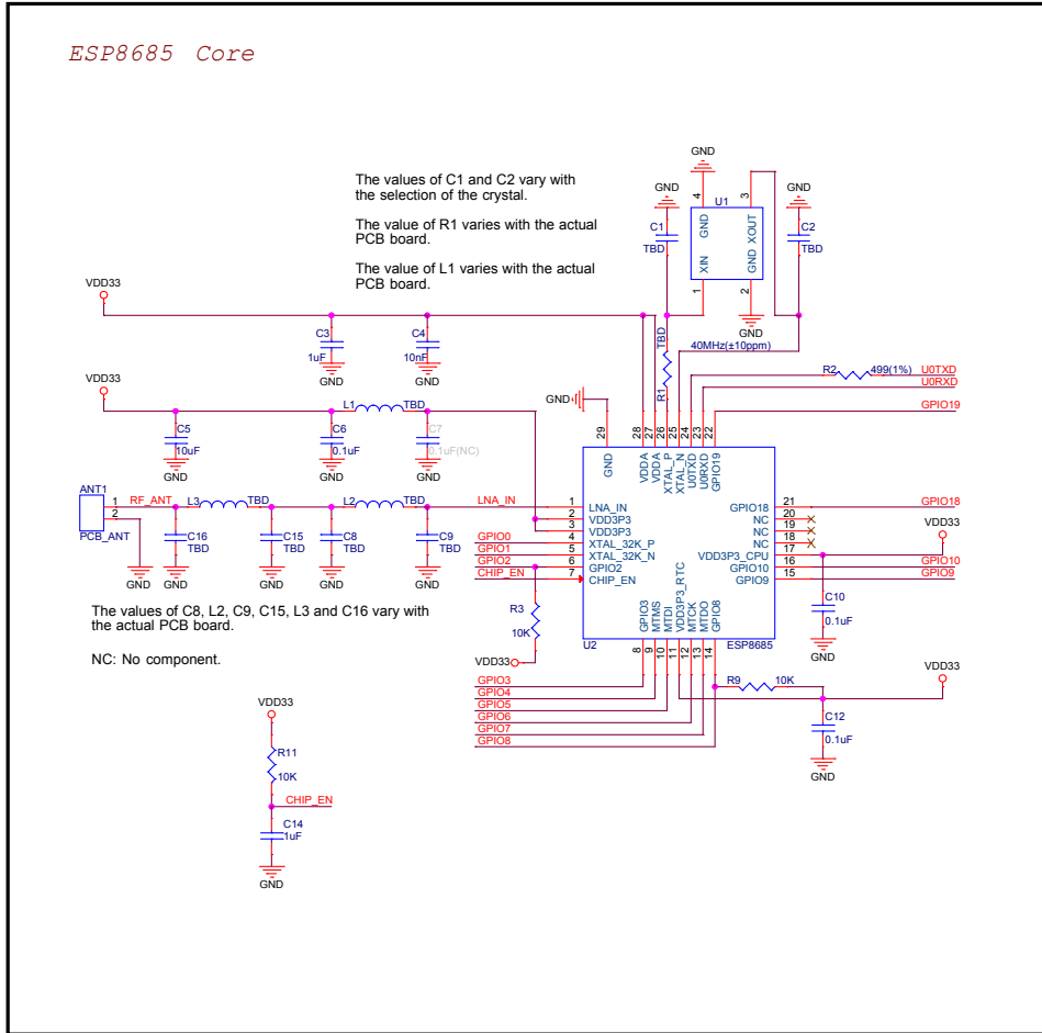
图 4: ESP8685-WROOM-06 原理图
