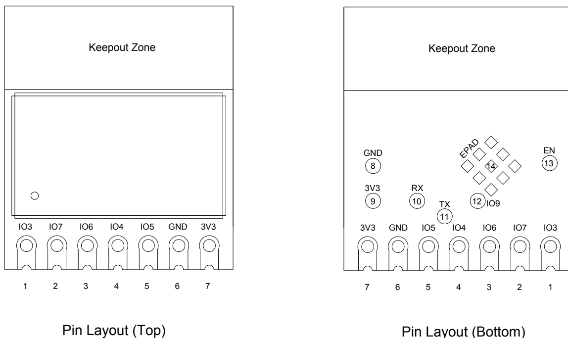
图 2: 管脚布局
