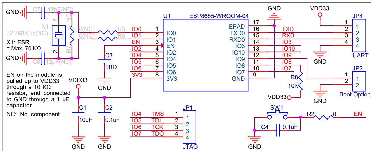
图 5: 外围设计原理图
