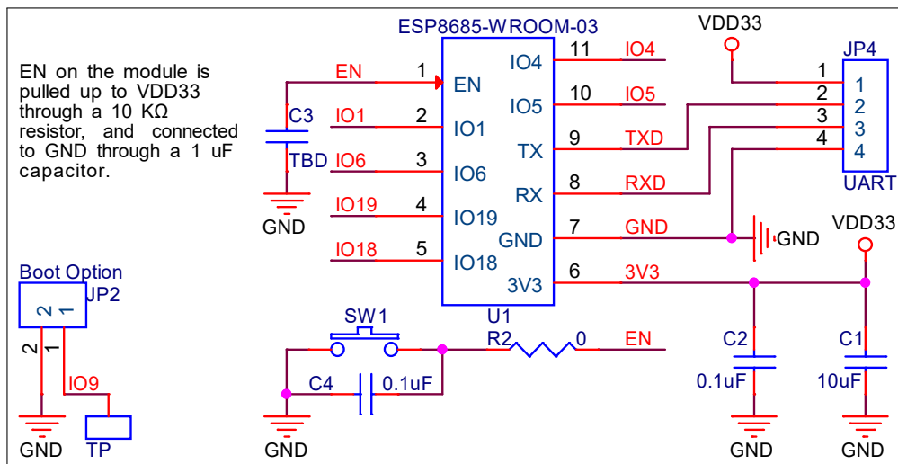
图 5: 外围设计原理图
