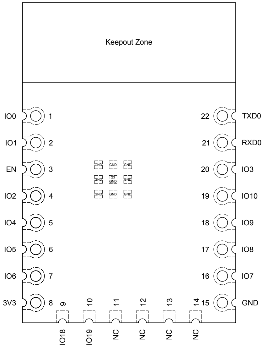
图 2: 管脚布局
