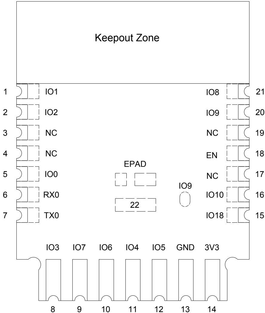
图 2: 管脚布局 (顶视图)
