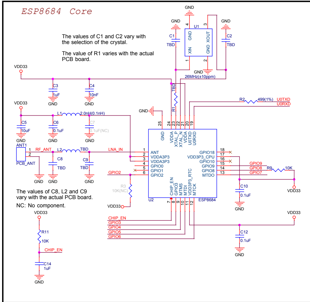
图 4: ESP8684-WROOM-05 原理图
