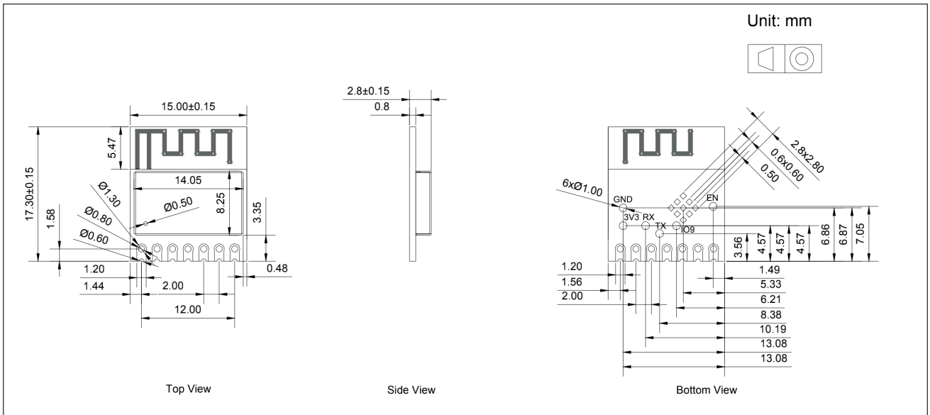
图 6: 模组尺寸
