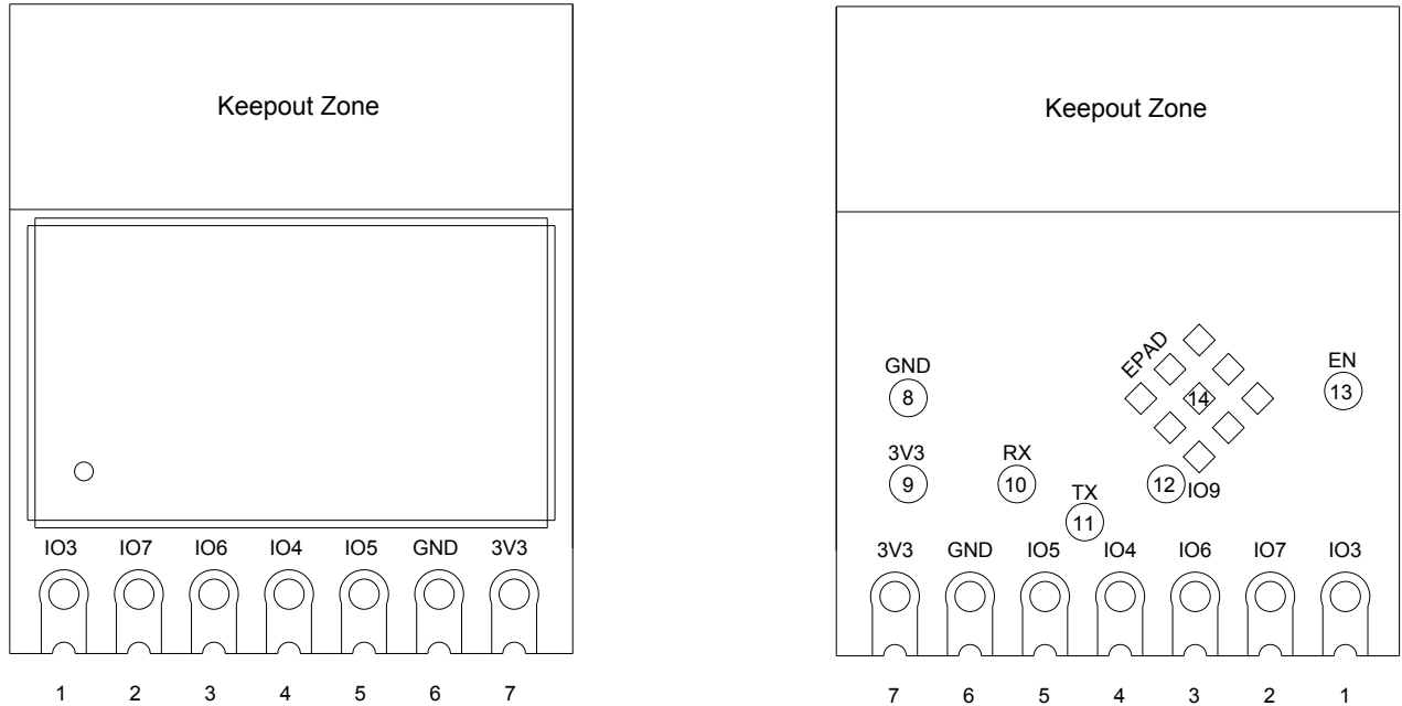
图 2: 管脚布局 (顶视图和底视图)
