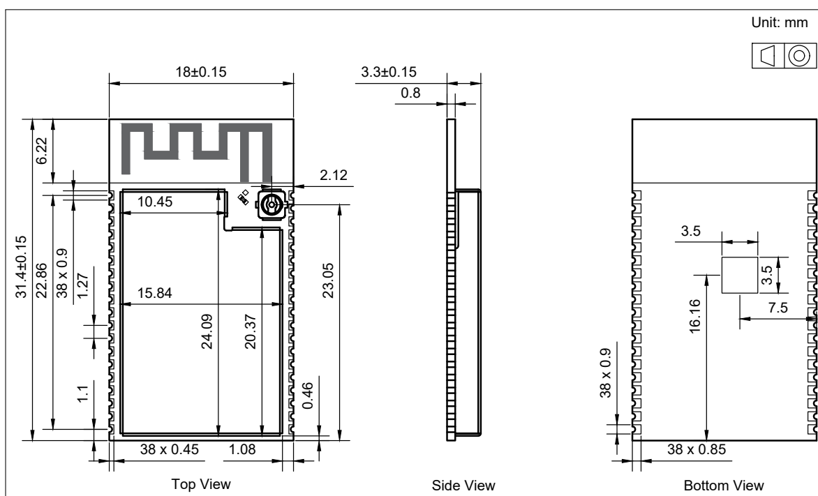
图 7: ESP32-WROVER-IB 模组尺寸
