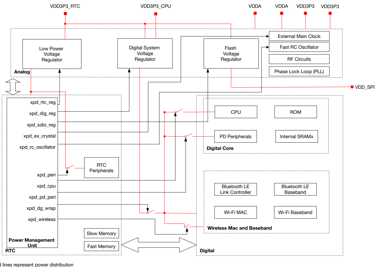
图 10-1. 低功耗管理原理图
