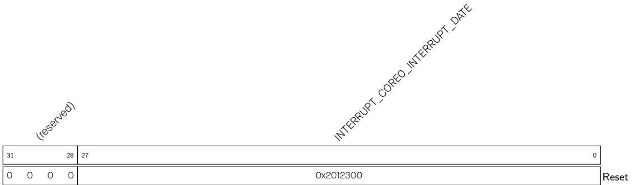
Register 9.90. INTERRUPT_CORE0_DATE_REG (0x07FC)
