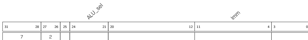
图 2-9. 指令类型 - 对阶段计数器寄存器的 ALU 运算
