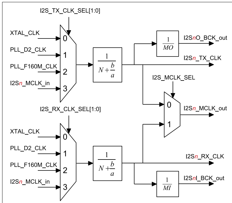
图 28-6. I2Sn 时钟
