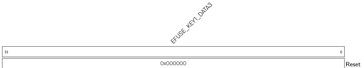
Register 5.51. EFUSE_RD_KEY1_DATA3_REG (0x00C8)
