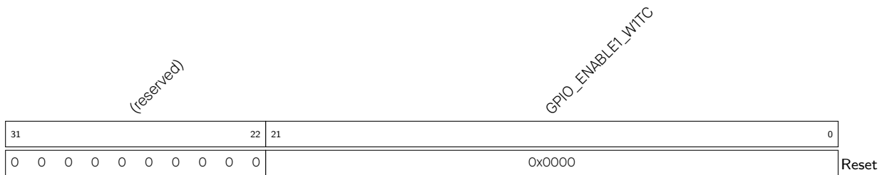
Register 6.14. GPIO_ENABLE1_W1TC_REG (0x0034)
