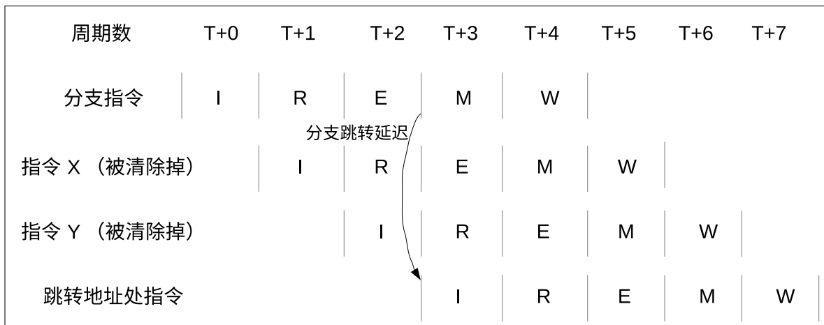
图 1-8. 控制冒险
