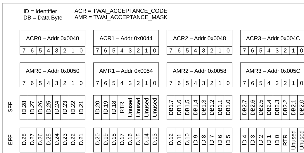
图 31-8. 单滤波模式
