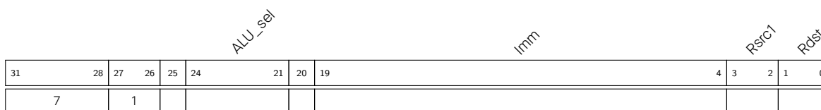
图 2-8. 指令类型 - 对指令立即值的 ALU 运算
