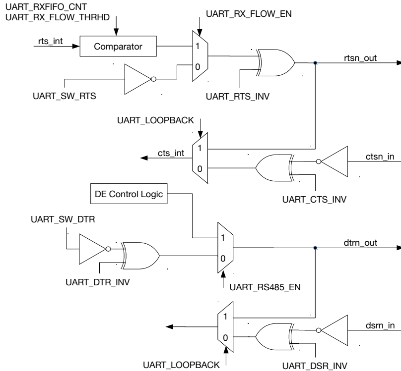
图 26-11. 硬件流控图
