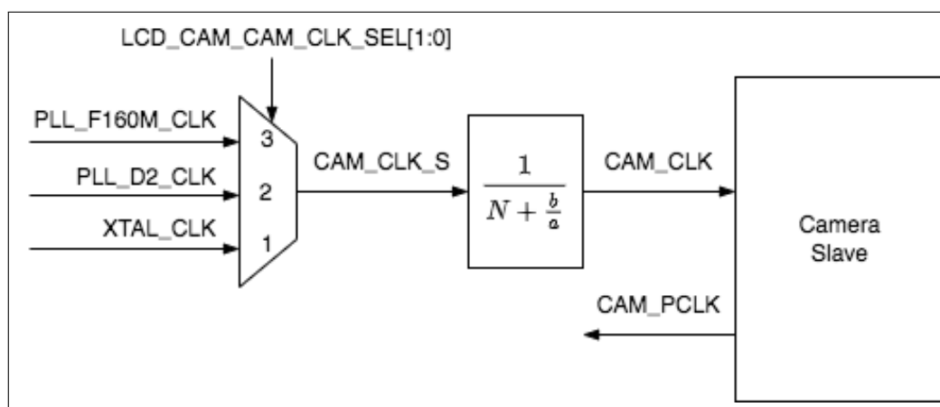
图 29-3. Camera 时钟
