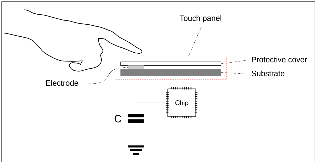
图 39-1. 触摸传感器
