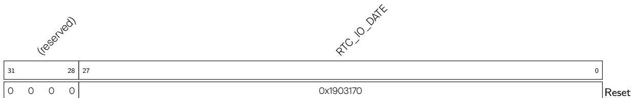
Register 6.58. RTC_IO_DATE_REG (0x01FC)
