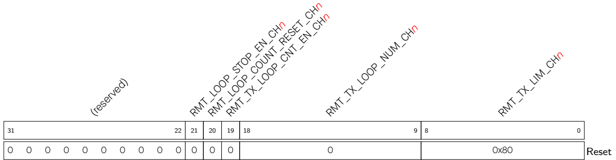
Register 3716. RMT_CH n _TX_LIM_REG ( n : 0-3) (0x00A0+0x4* n )
