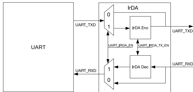
图 26-10. IrDA 编解码结构图
