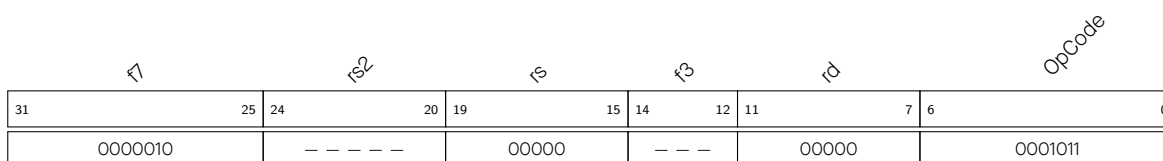
图 2-29. 中断指令 - retirq
