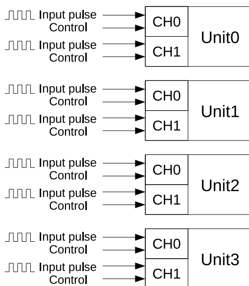
图 38-1. PCNT 框图
