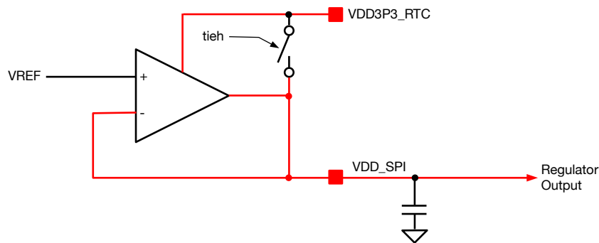
图 10-7. Flash 调压器
