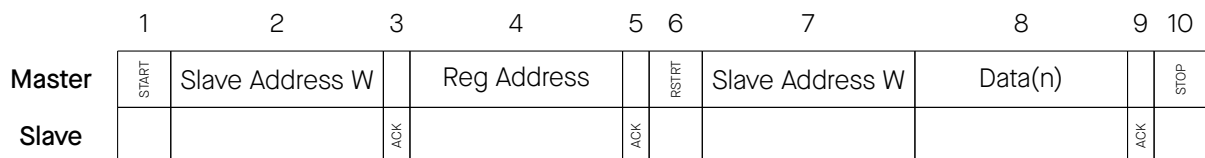
图 2-32. I2C 写操作
