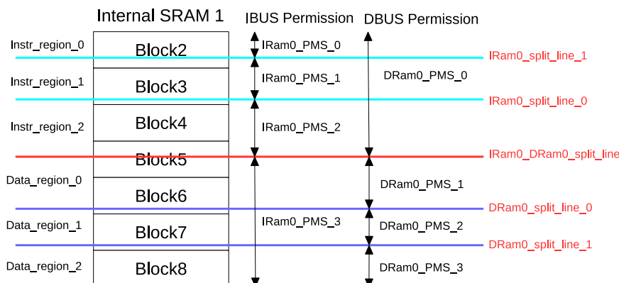
图 15-1. Internal SRAM1 的区域分割示意图
