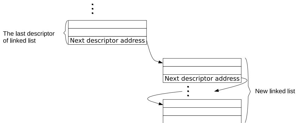
图 3-5. 链表关系图
