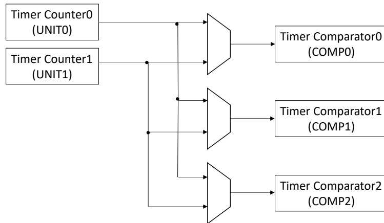
图 11-1. 系统定时器结构图
