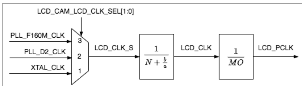
图 29-2. LCD 时钟
