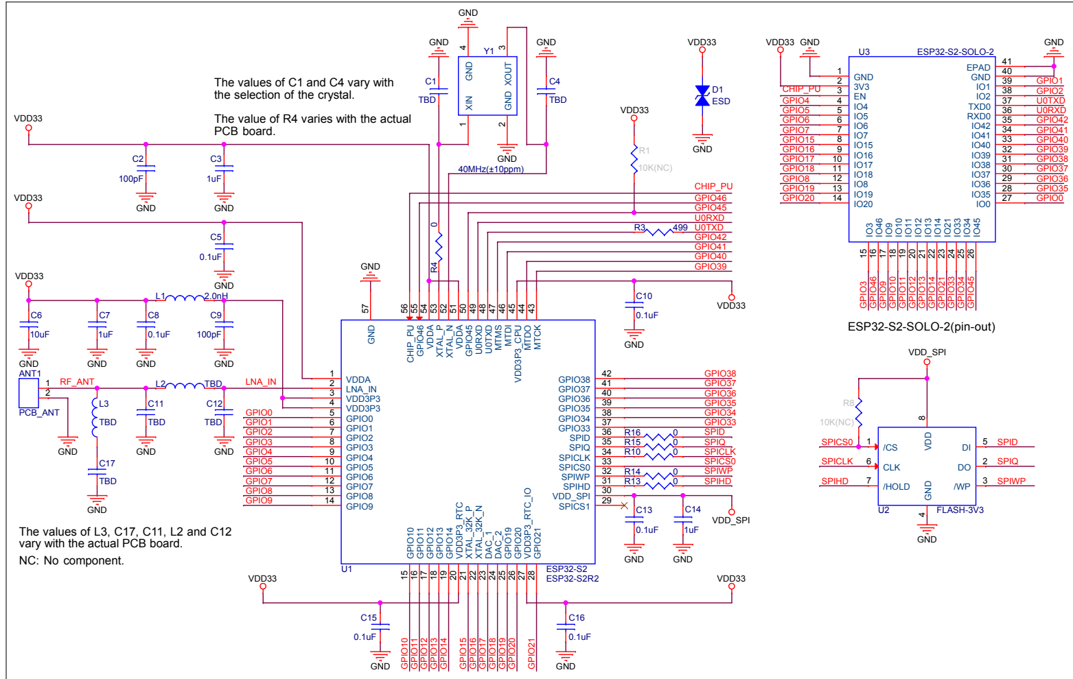
图 5: ESP32-S2-SOLO-2 原理图
