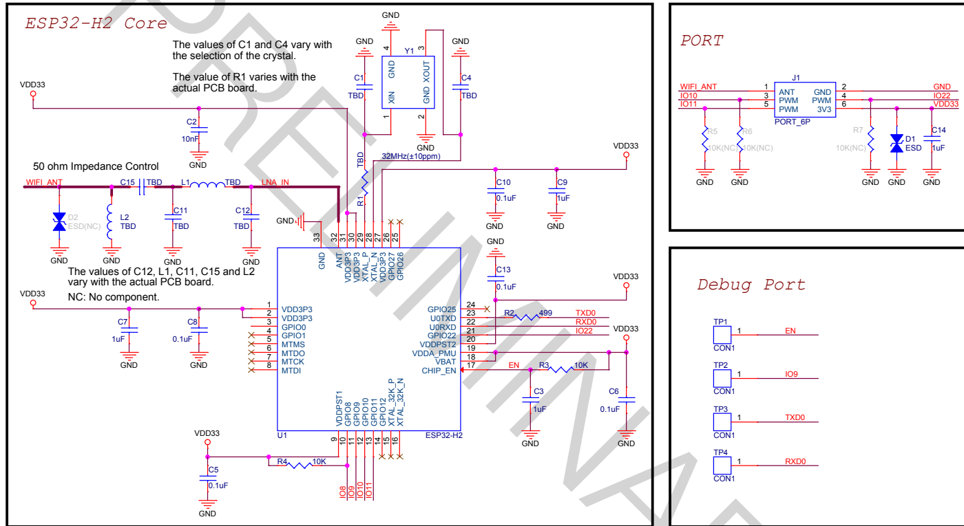
图 4: 原理图
