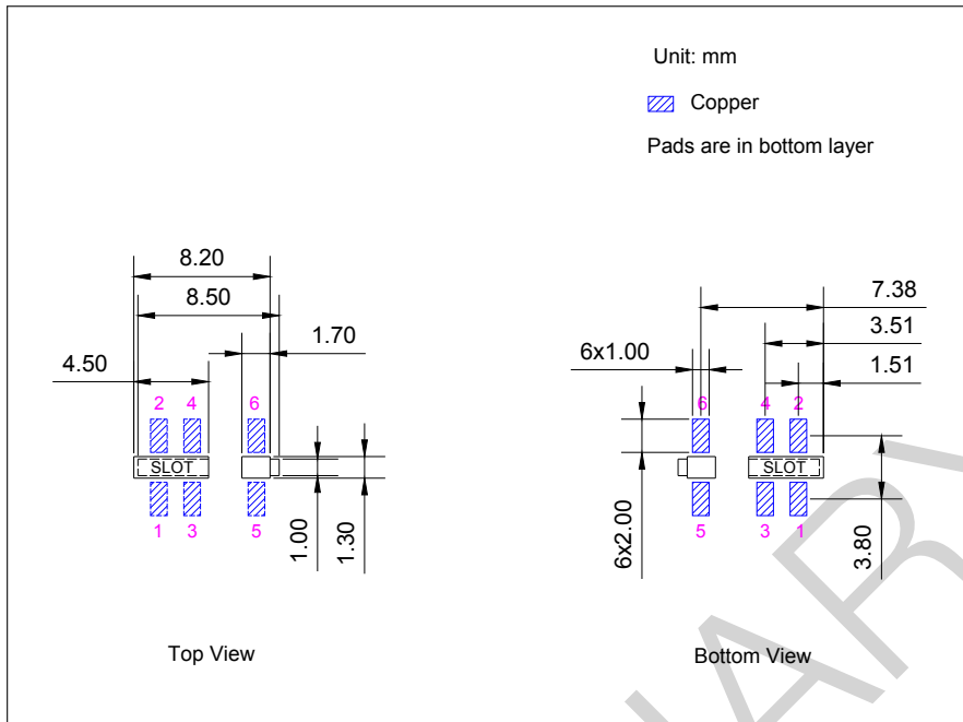
图 7: 推荐 PCB 封装图形
