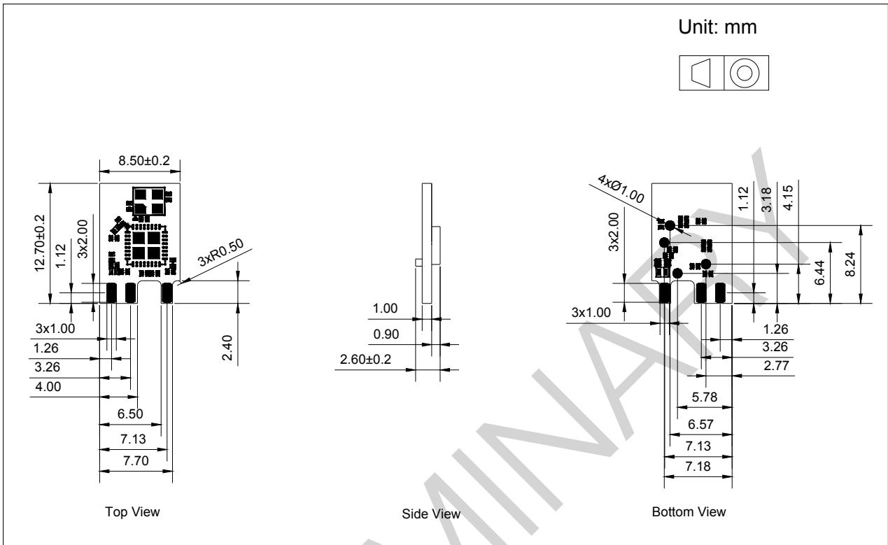
图 6: 模组尺寸
