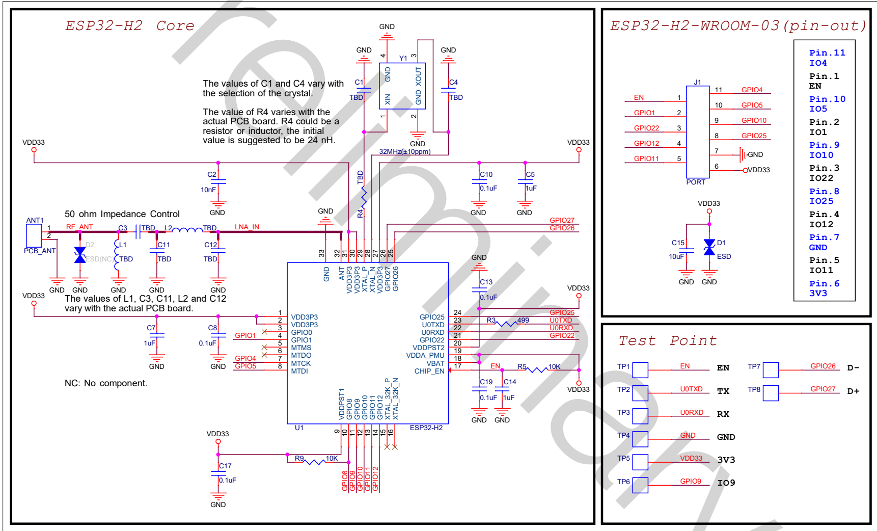
图 4: 原理图
