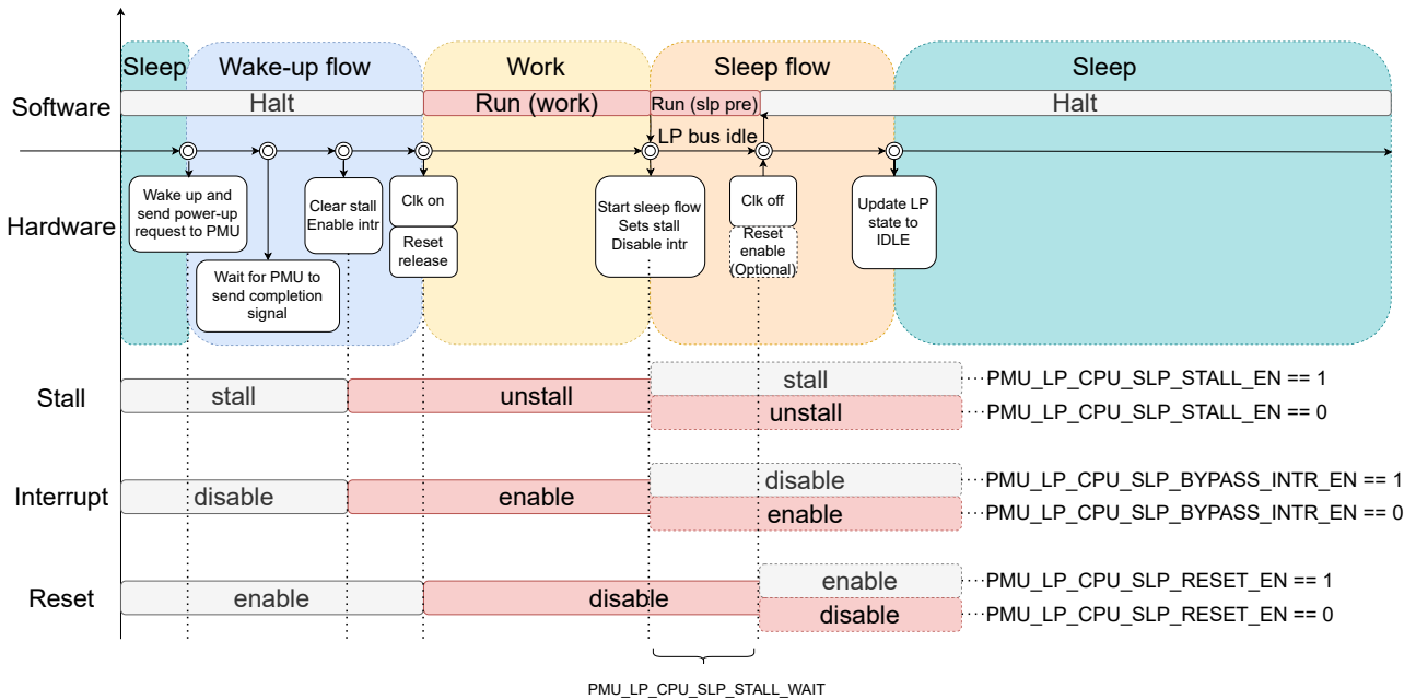
图 3-2. LP CPU 唤醒和睡眠流程
