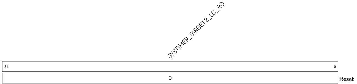
Register 12.34. SYSTIMER_REAL_TARGET2_LO_REG (0x0084)
