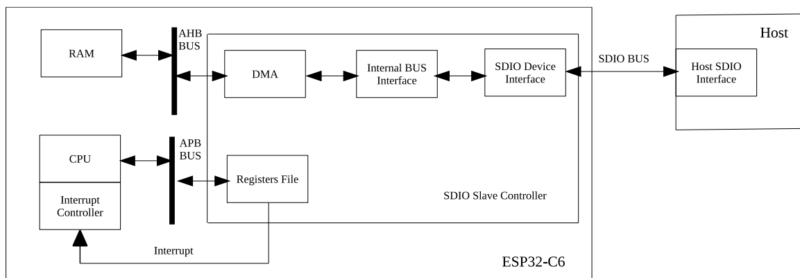
图 33-1. SDIO 从机功能结构图
