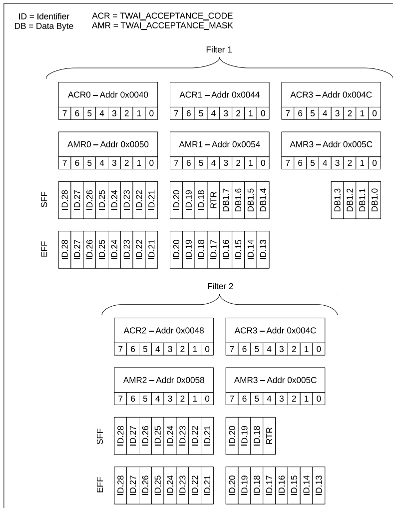
图 32-9. 双滤波模式
