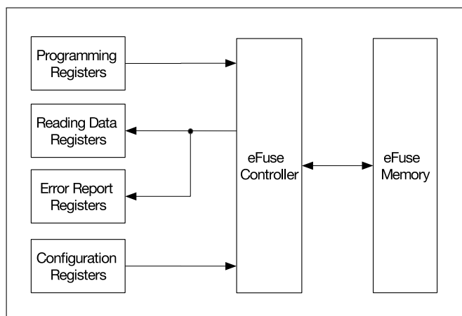
图 6-1. eFuse 系统数据通路
