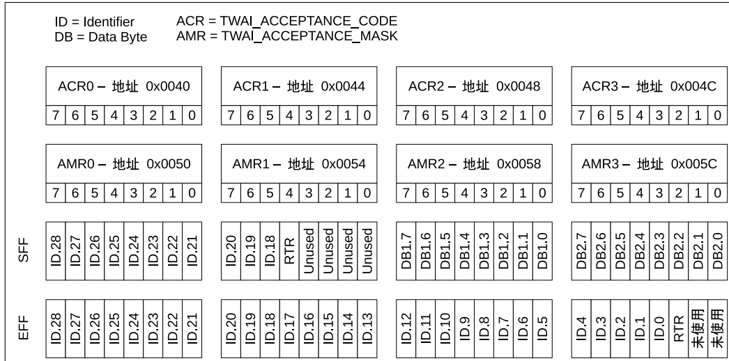
图 32-8. 单滤波模式
