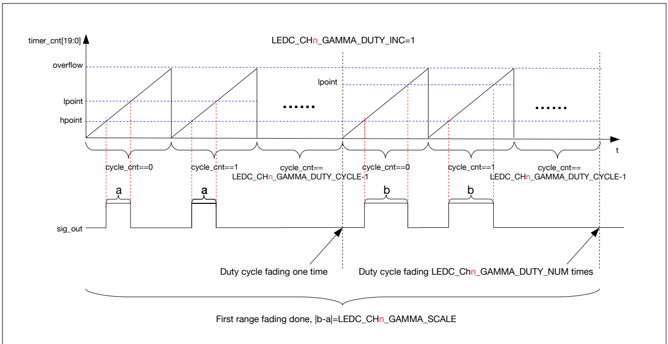
图 34-6. 输出信号占空比线性渐变图
