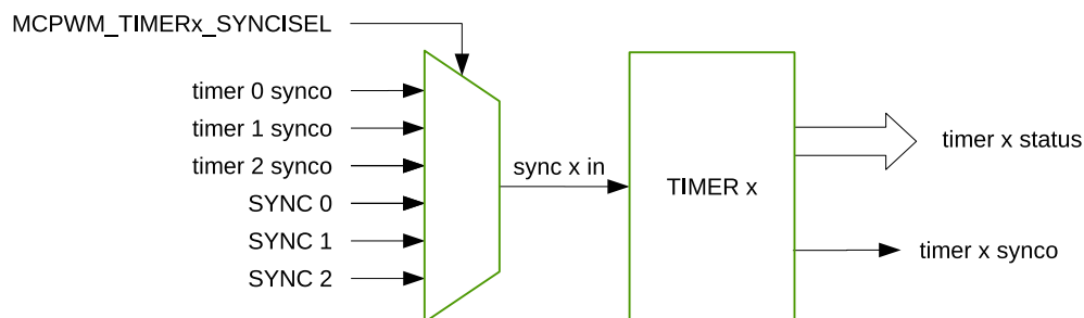
图 35-3. 定时器模块
