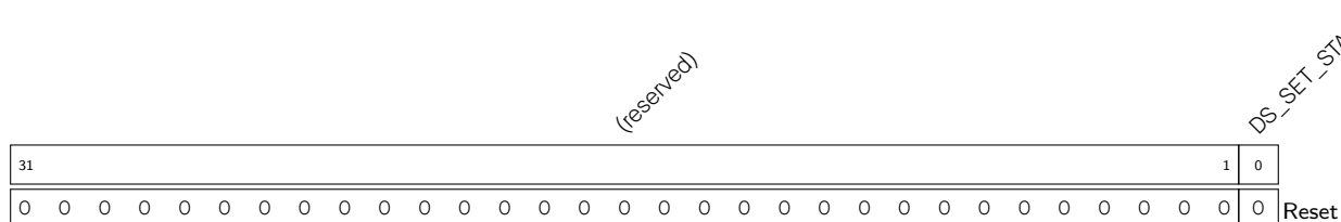
Register 23.2. DS_SET_START_REG (0x0E00)
