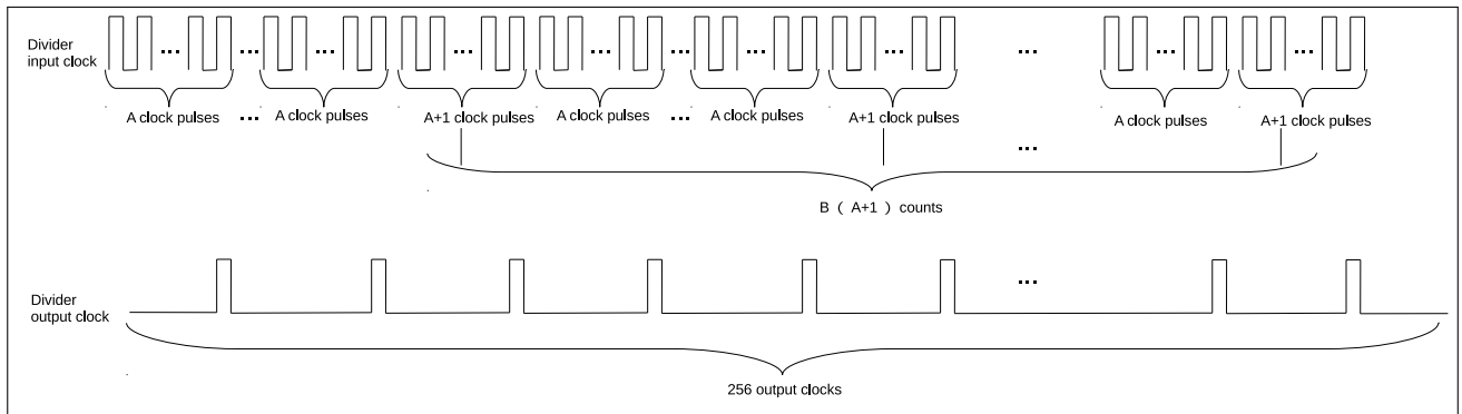
图 34-3. LEDC_CLK_DIV 非整数时的分频
