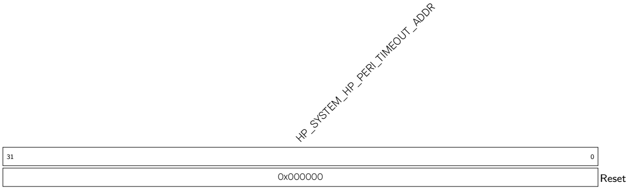
Register 16.8. HP_SYSTEM_HP_PERI_TIMEOUT_ADDR_REG (0x001C)
