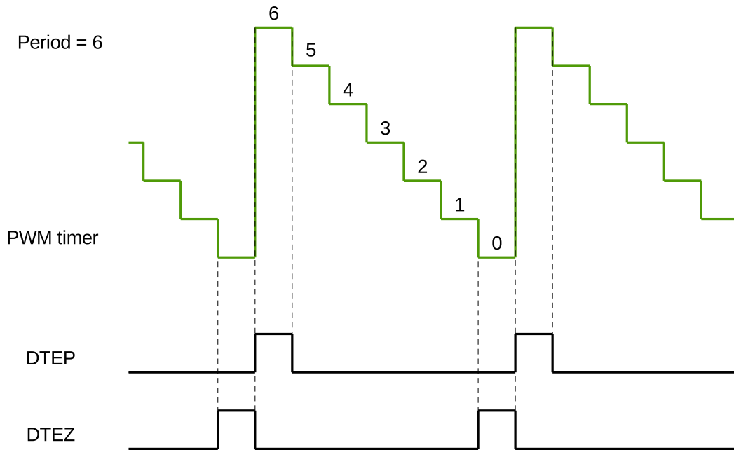
图 35-13. 递减模式中生成的 DTEP 和 DTEZ
