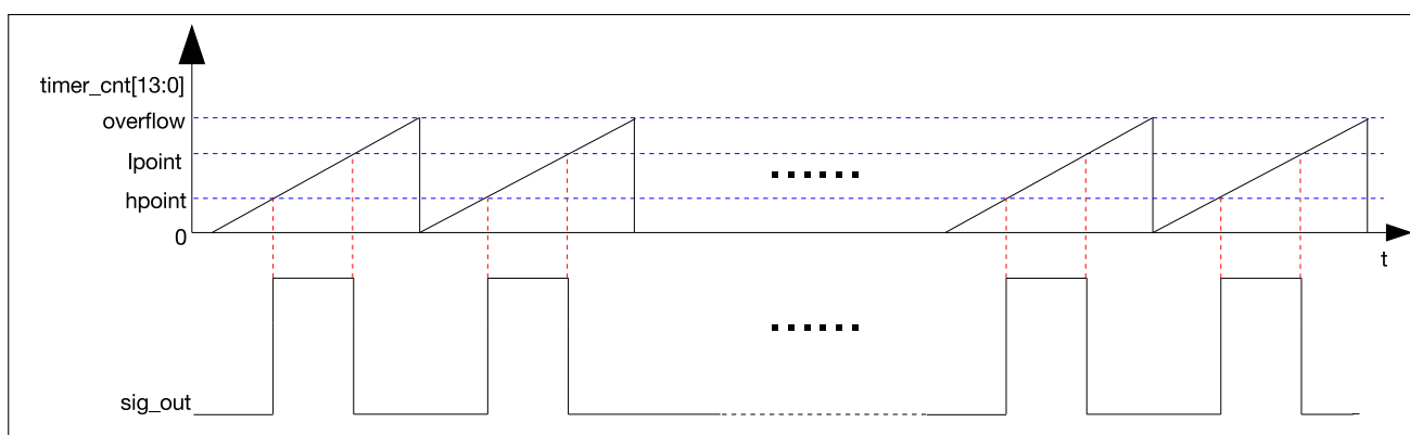
图 34-5. LED PWM 输出信号图
