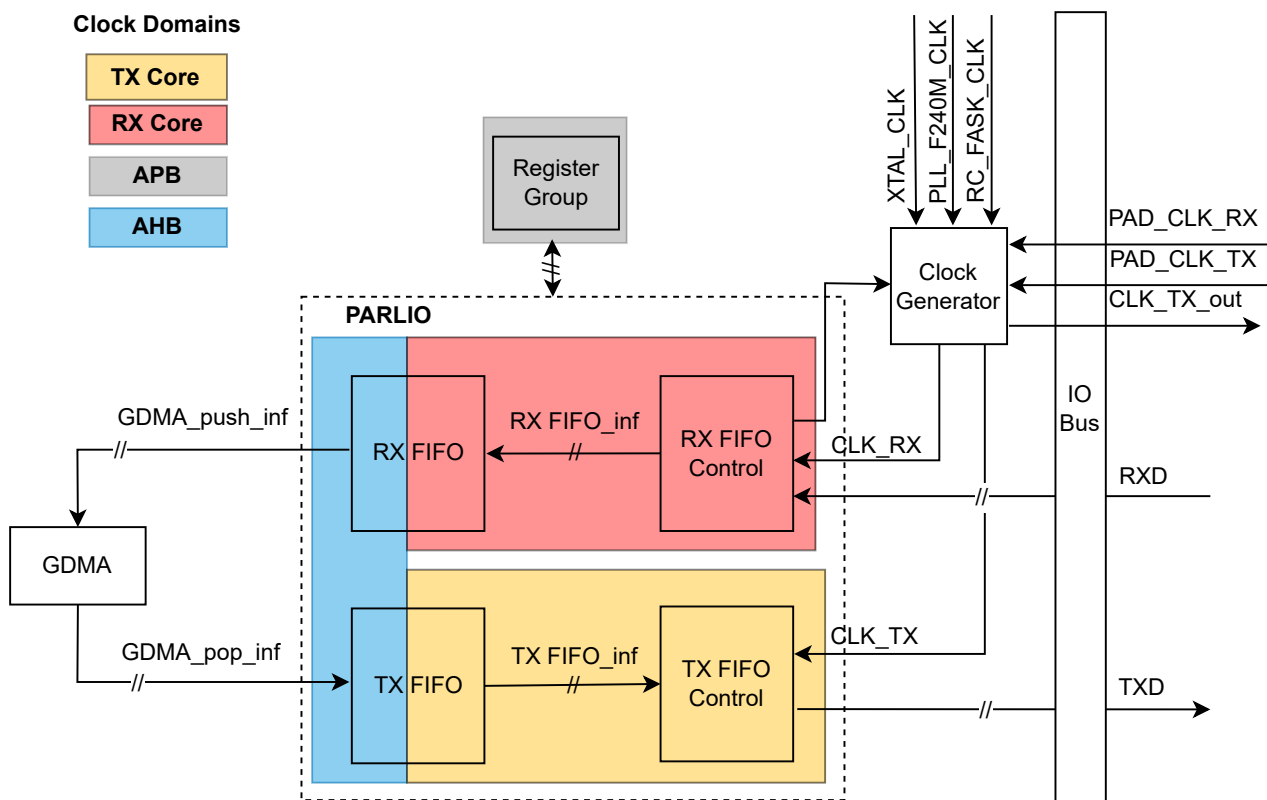
图 37-1. PARLIO 系统框图
