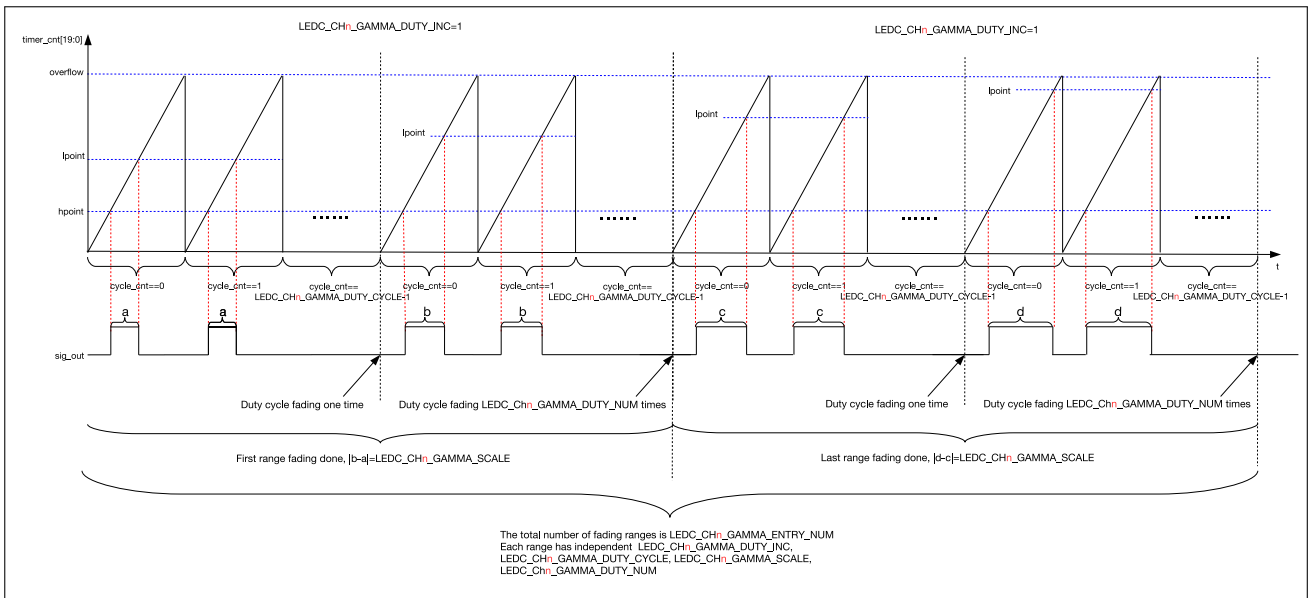
图 34-7. 输出信号占空比伽玛曲线渐变图
