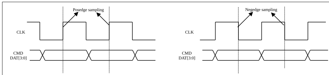
图 33-9. 采样时序图
