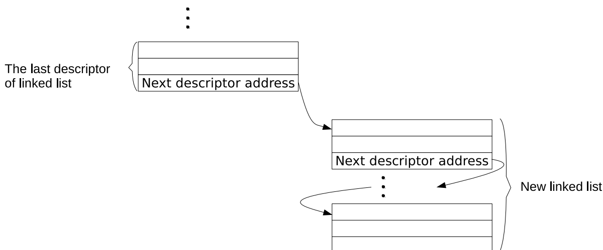
图 4-4. 链表关系图
