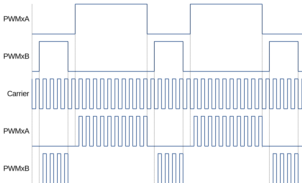
图 35-29. PWM 载波操作的波形示例
