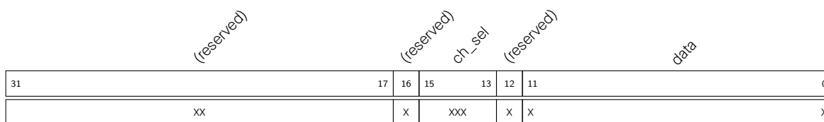
图 38-8. DMA 数据格式
