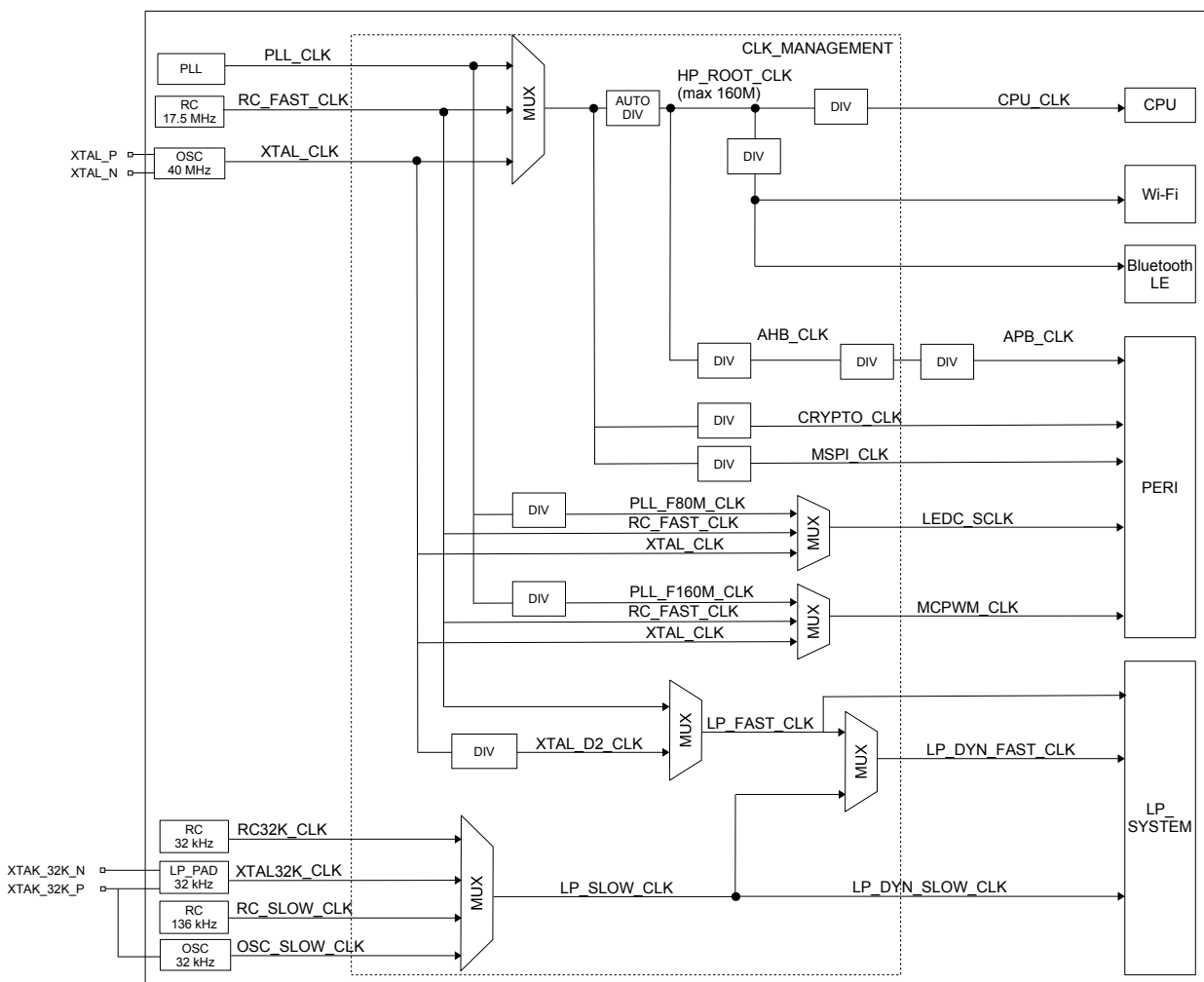
图 8-2. 系统时钟
