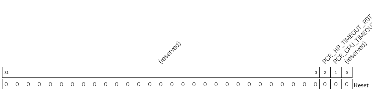
Register 8.62. PCR_TIMEOUT_CONF_REG (0x010C)
