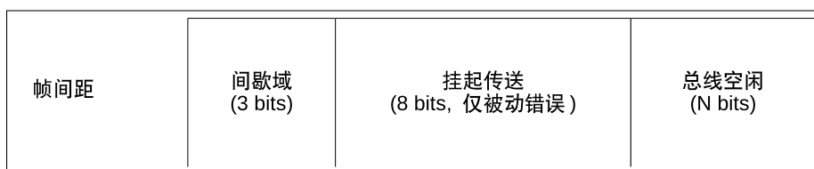
图 32-4. 帧间距中的域
