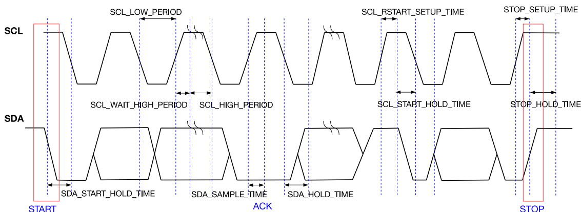
图 28-5. I2C 时序图
