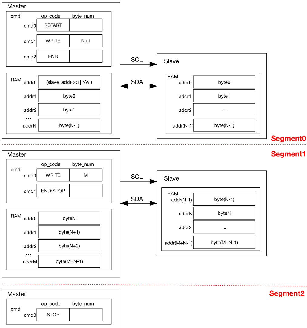
图 28-10. I2C 主机分段写 7 位寻址的从机
