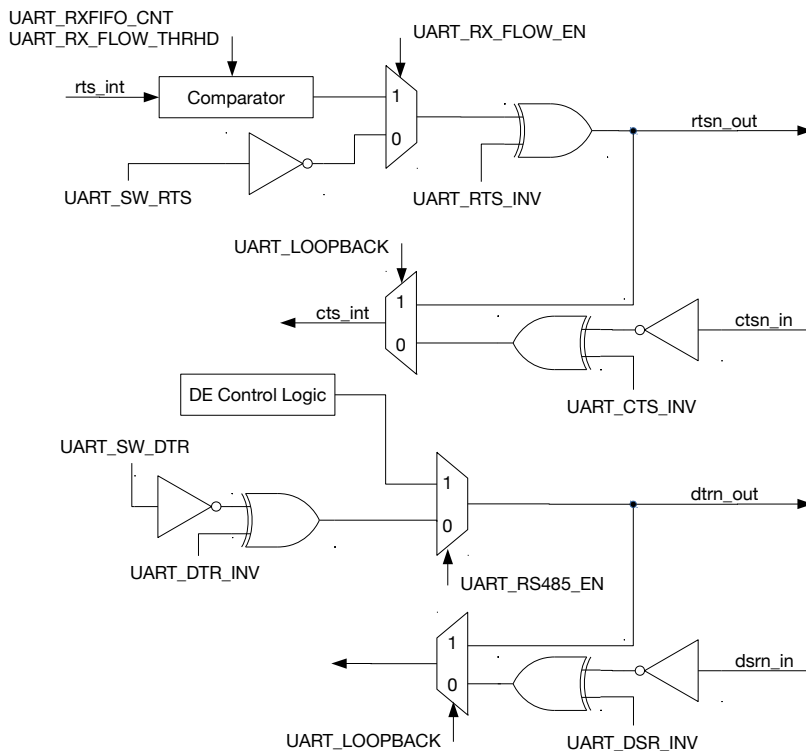
图 26-9. 硬件流控图
