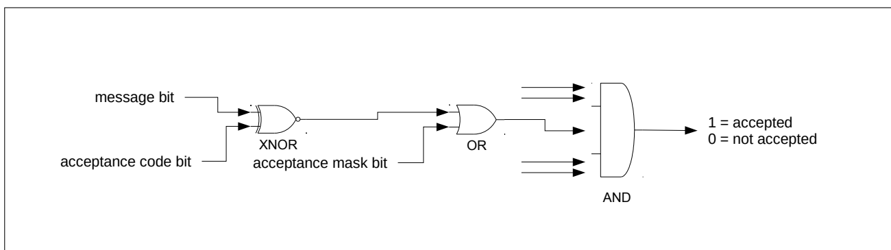
图 32-7. 接收滤波器
