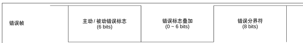
图 32-2. 错误帧中的位域
