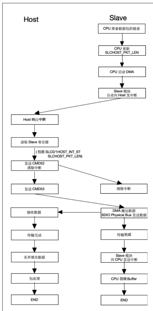
图 33-11. 从机向主机发送包的流程
