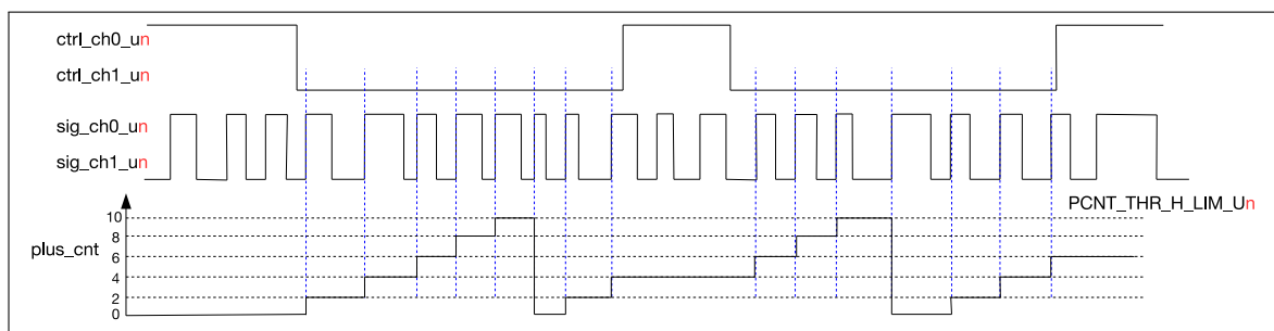
图 30-5. 双通道递增计数图
