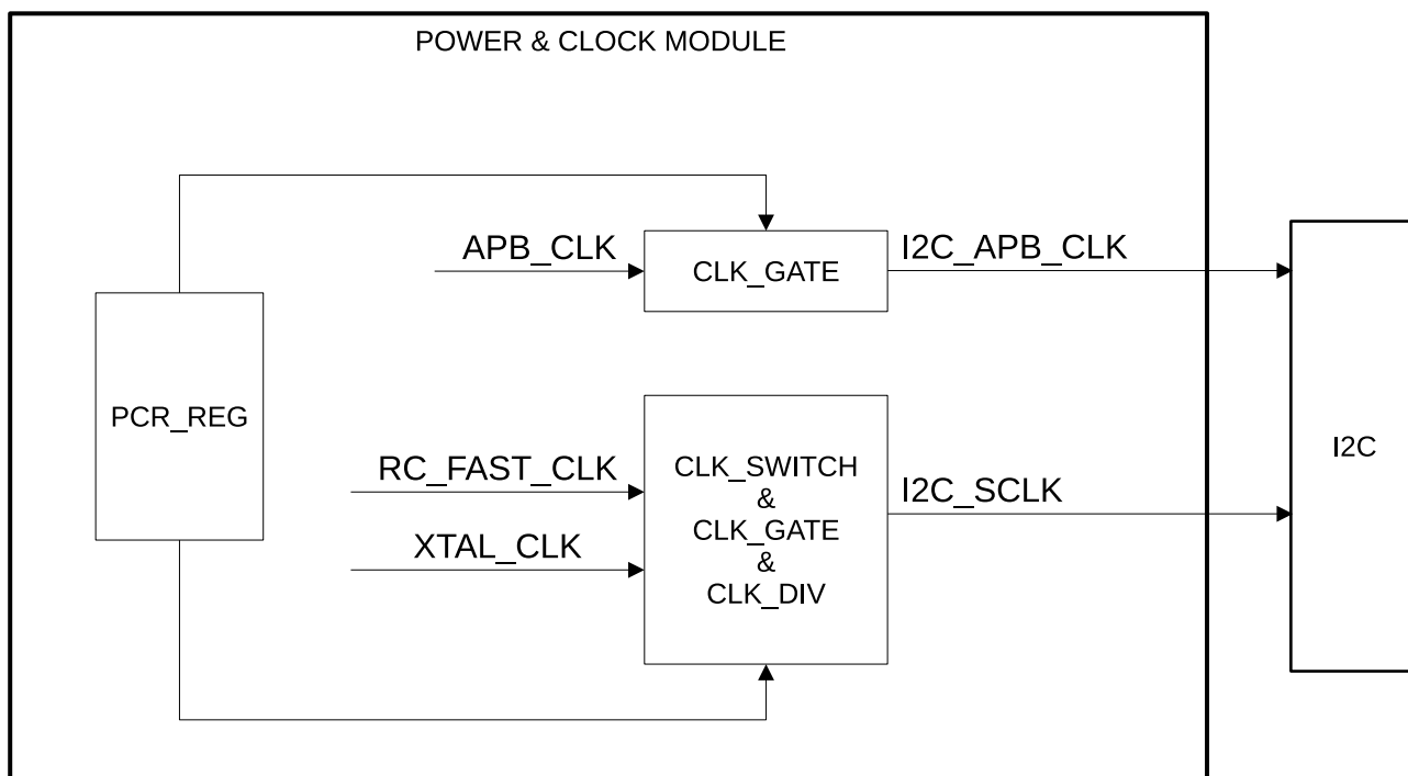
图 8-3. 时钟配置示例
