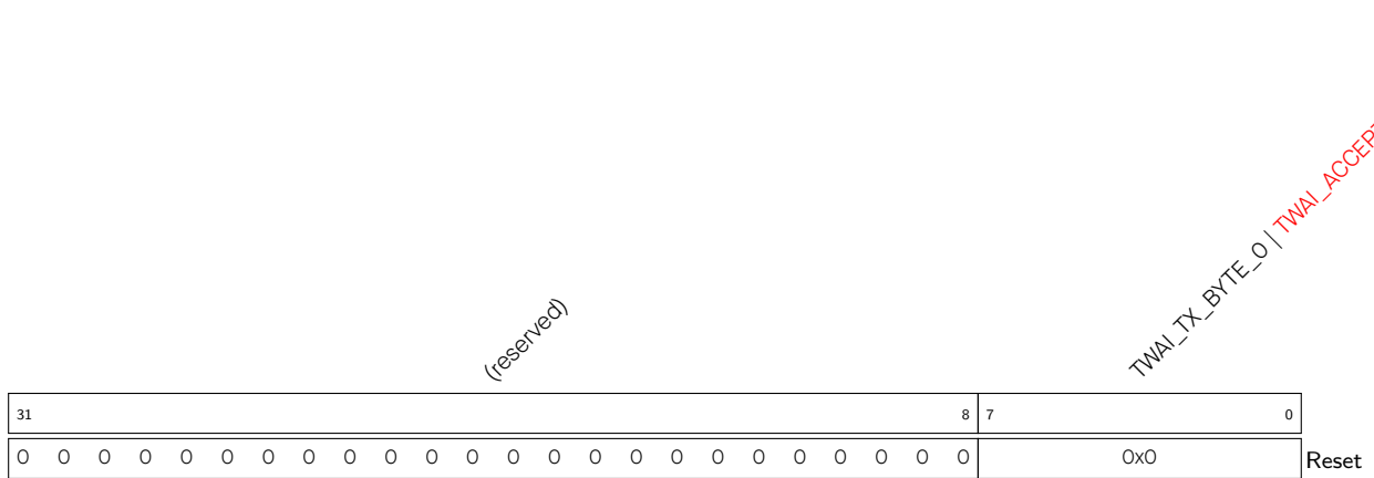
Register 32.5. TWAI_DATA_0_REG (0x0040)
