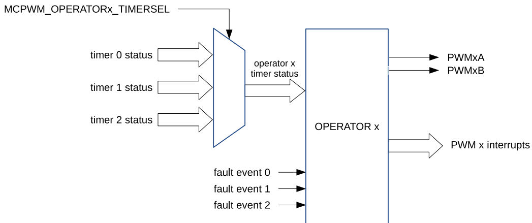
图 35-4. 操作器模块
