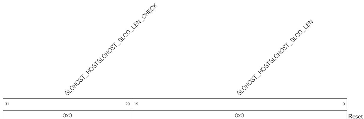
Register 33.51. SLCHOST_PKT_LEN_REG (0x0060)
