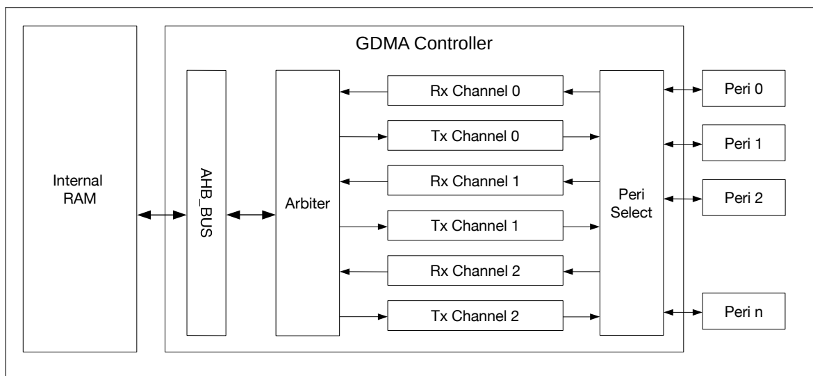
图 4-2. GDMA 控制器的架构
