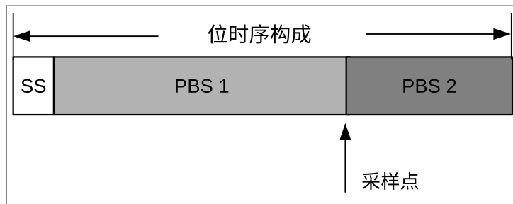
图 32-5. 标称位构成
