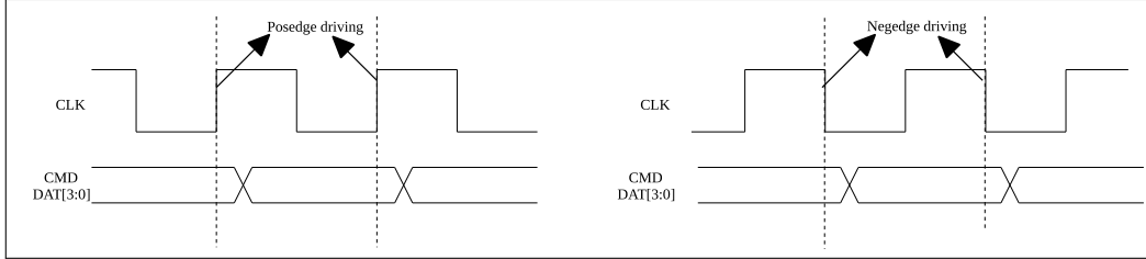
图 33-10. 输出时序图
