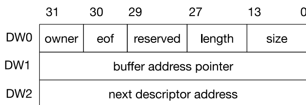
图 33-6. SDIO 从机 DMA 链表描述符结构
