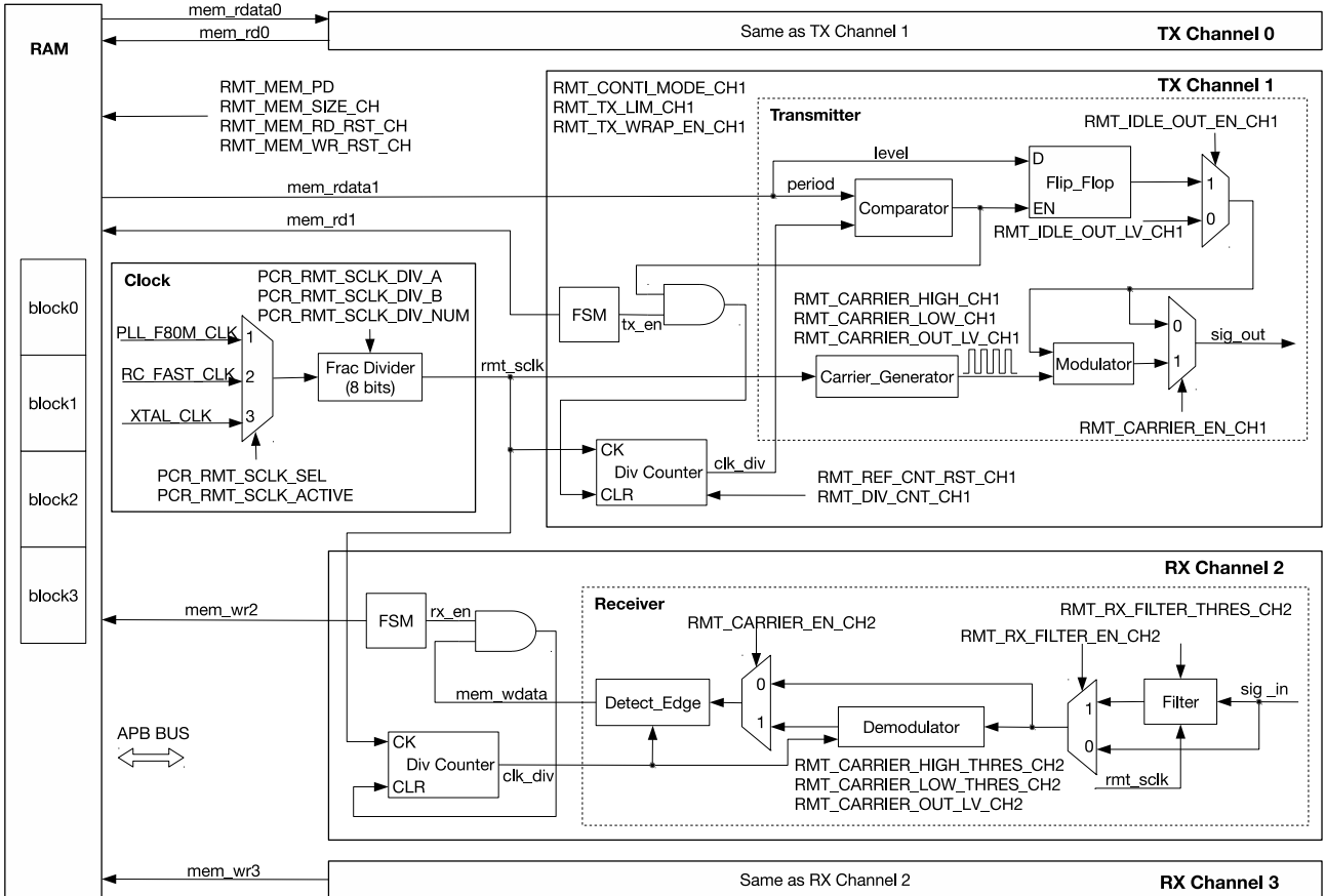
图 36-1. RMT 结构框图
