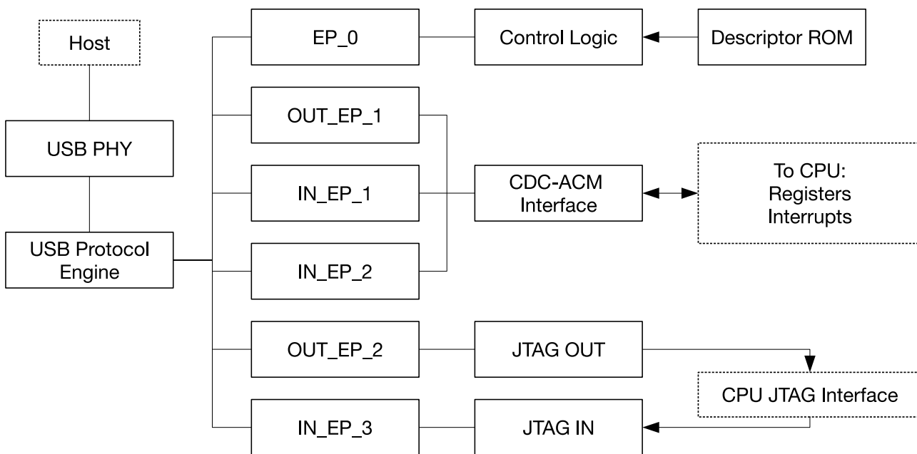
图 31-2. USB 串口/JTAG 控制器框图
