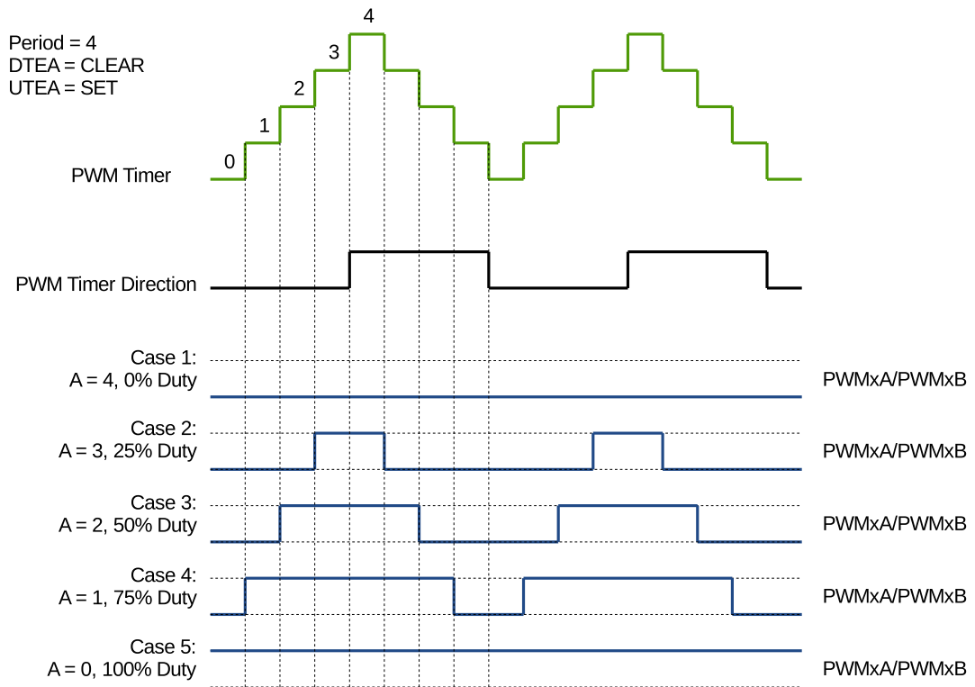
图 35-16. 递增递减模式下的对称波形
