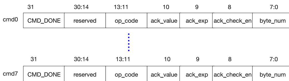
图 28-6. I2C 命令寄存器结构
