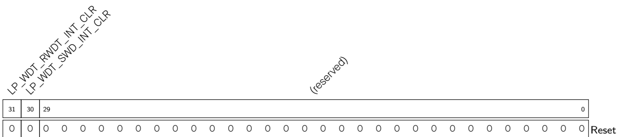
Register 14.13. LP_WDT_RWDT_INT_CLR_REG (0x0030)
