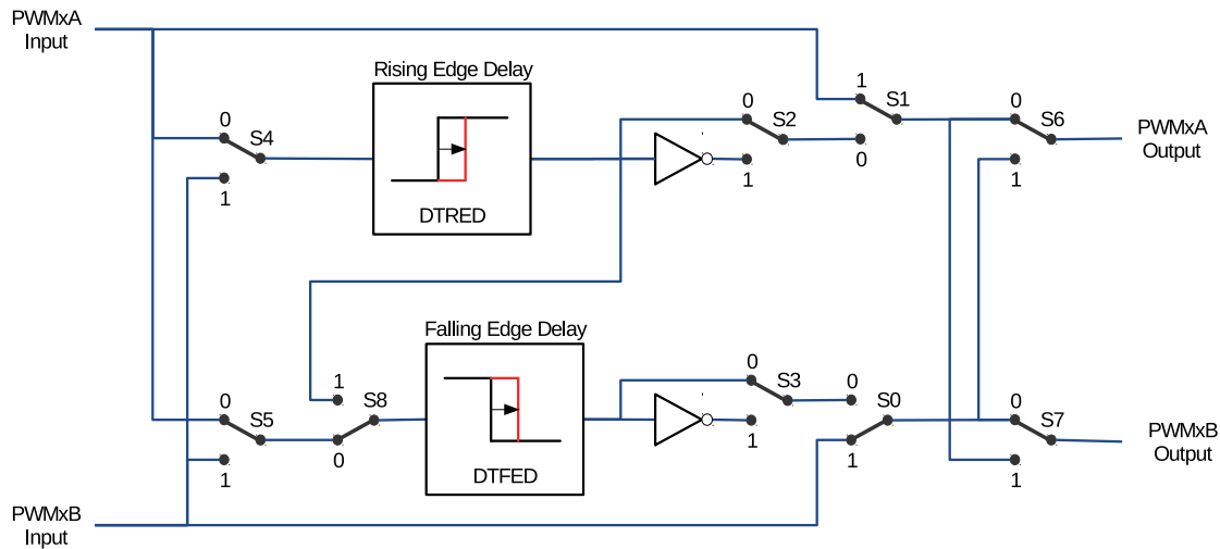
图 35-24. 死区模块的开关拓扑
