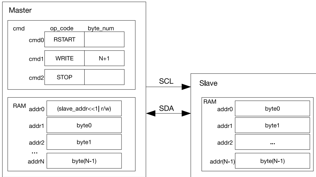
图 28-7. I2C 主机写 7 位寻址的从机
