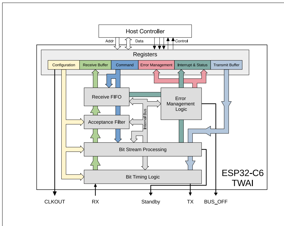
图 32-6. TWAI 概略图
