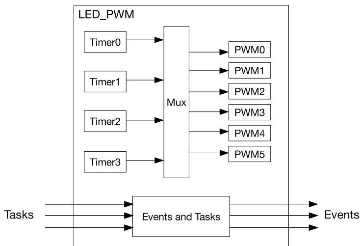
图 34-1. LED PWM 控制器架构
