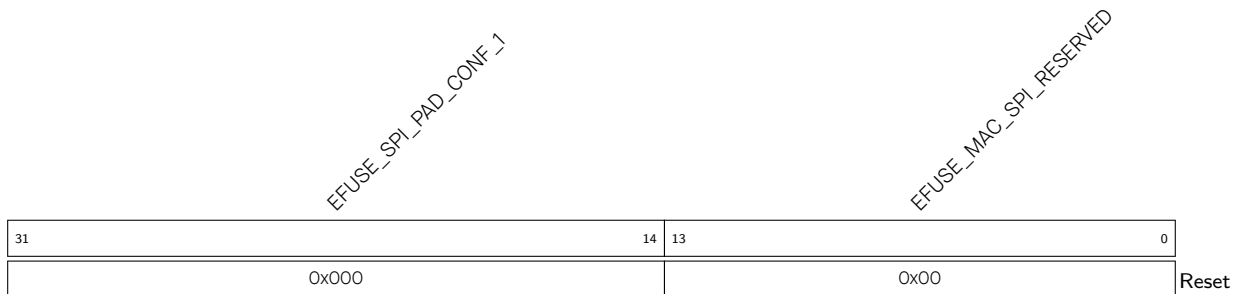
Register 6.20. EFUSE_RD_MAC_SPI_SYS_2_REG (0x004C)
