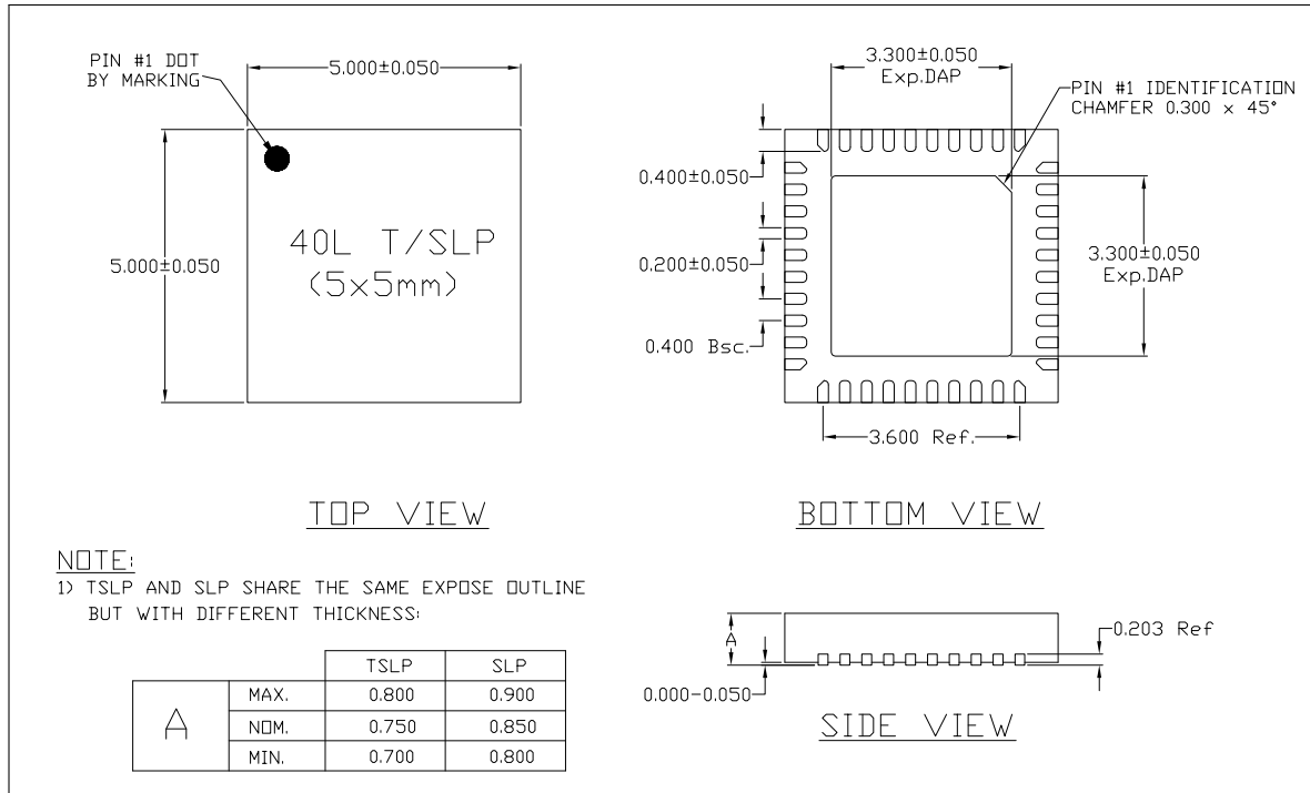
图 7-1. QFN40 (5x5 mm) 封装
