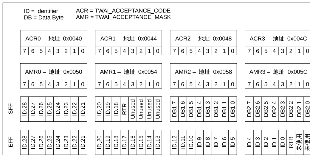
图 31-8. 单滤波模式
