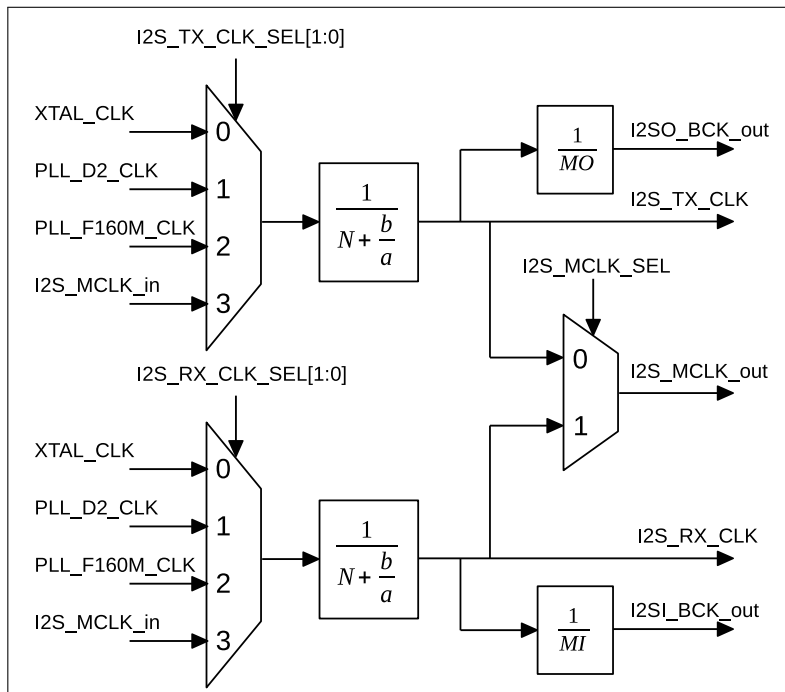
图 29-6. I2S 时钟
