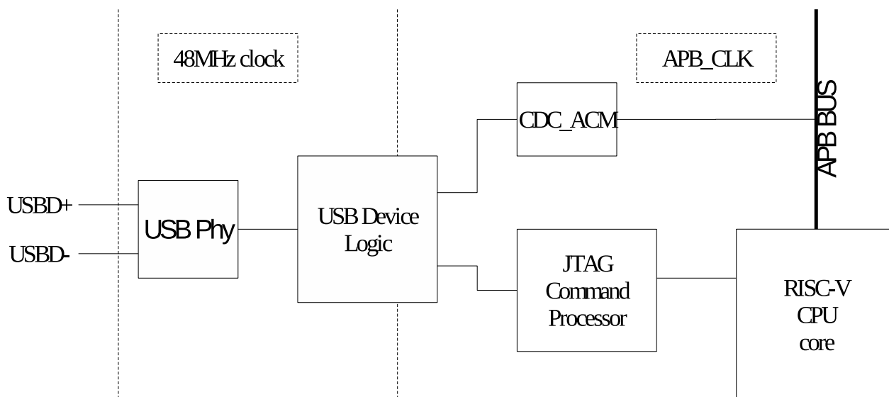
图 30-1. USB Serial/JTAG 高层框图
