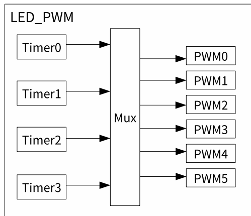
图 32-1. LED PWM 控制器架构
