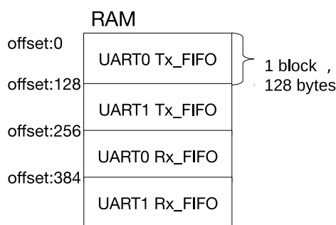
图 26-3. UART 共享 RAM 图
