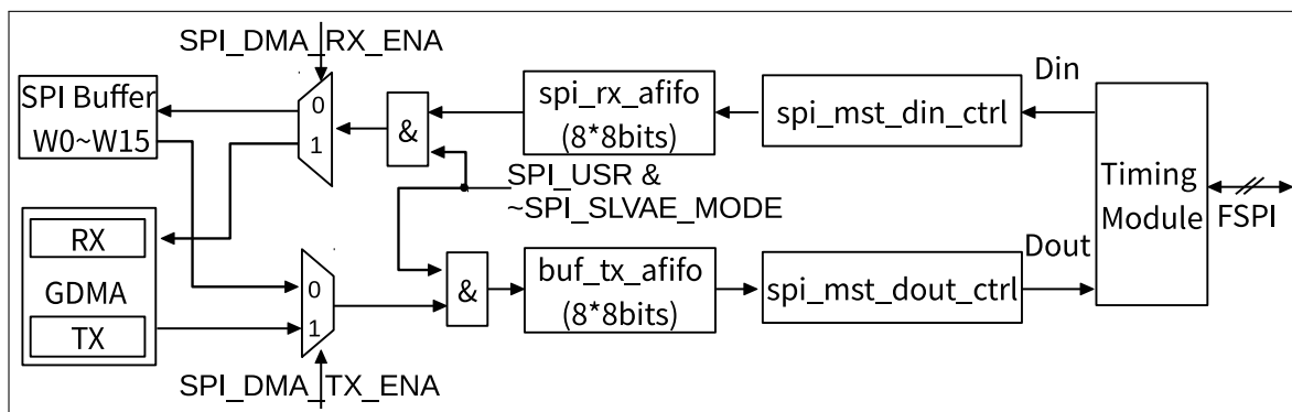
图 27-4. GP-SPI2 主机模式下的数据流控制
