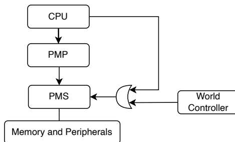
图 14-1. Permission Control Overview
