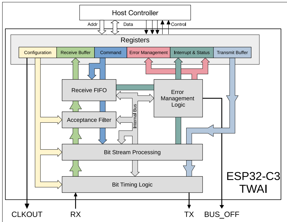
图 31-6. TWAI 概略图
