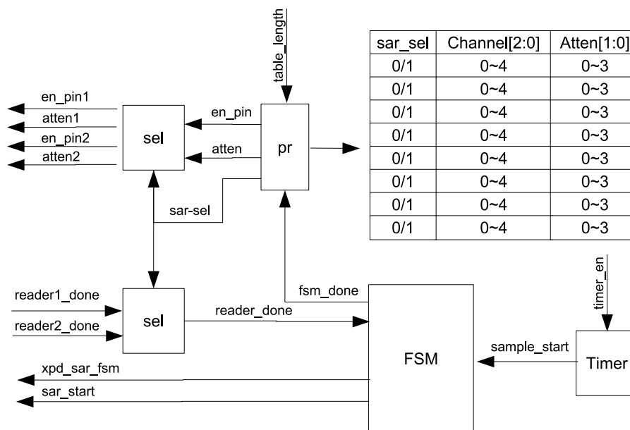
图 34-2. DIG ADC FSM 概况
