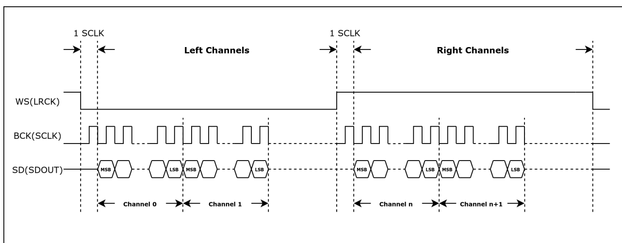
图 29-2. 时序图 - TDM Philips 标准
