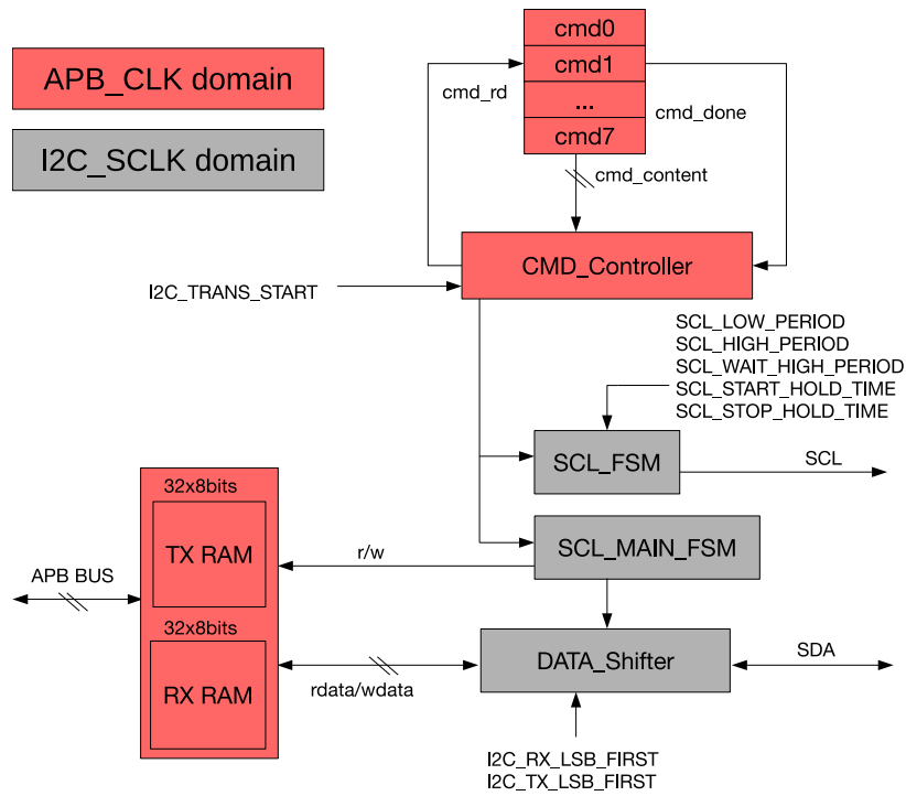
图 28-1. I2C 主机基本架构
