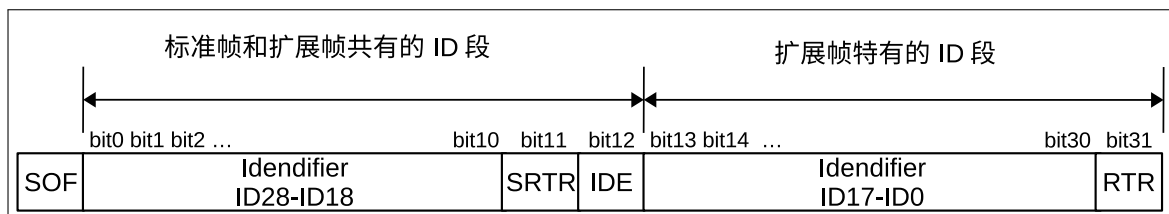
图 31-11. 丢失仲裁的 bit 位置
