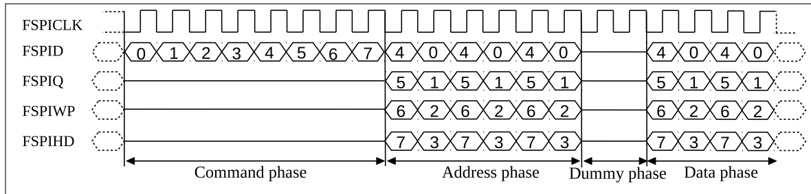
图 27-9. GP-SPI2 发送到 Flash 的 SPI Quad I/O 命令序列
