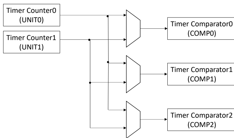
图 10-1. 系统定时器结构图
