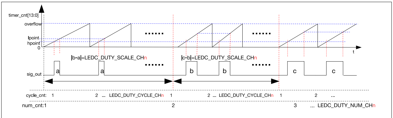
图 32-5. 输出信号占空比渐变图
