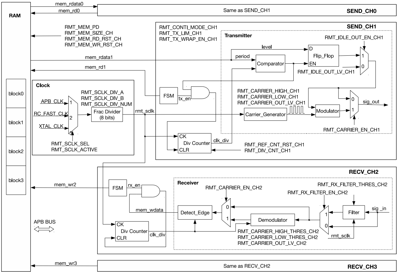
图 33-1. RMT 结构框图
