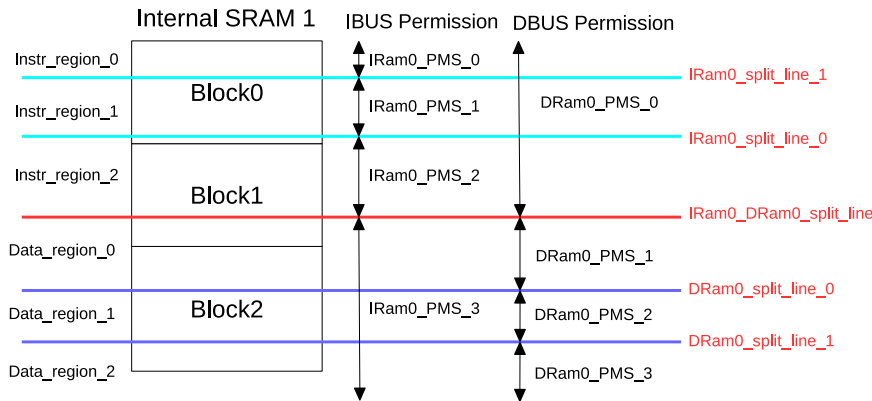
图 14-2. Internal SRAM1 的区域分割示意图
