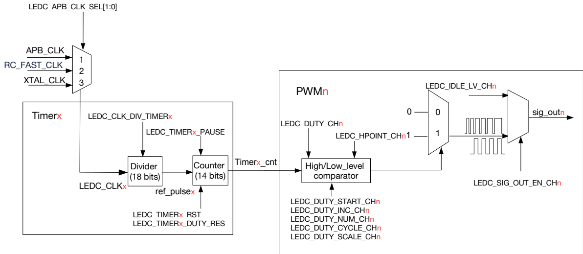
图 32-2. 定时器和 PWM 生成器功能块
