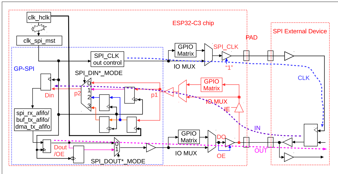
图 27-15. GP-SPI2 主机模式下时序补偿控制图
