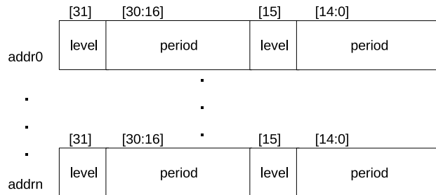
图 33-2. RAM 中脉冲编码结构
