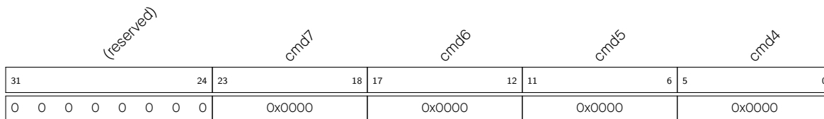
图 34-4. APB_SARADC_SAR_PATT_TAB2_REG 与样式 4 - 7
