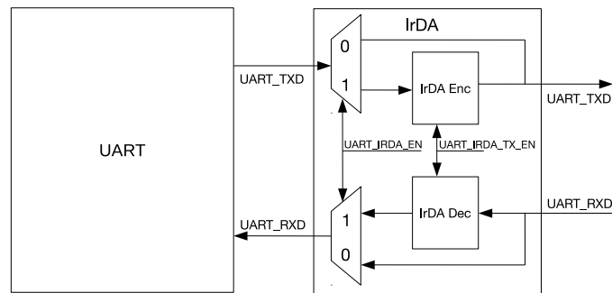
图 26-10. IrDA 编解码结构图
