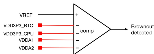
图 9-7. 欠压检测器
