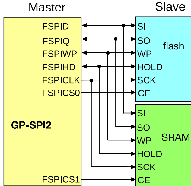
图 27-8. 4-bit 模式下 GP-SPI2 与 Flash 以及外部 RAM 的连接方式
