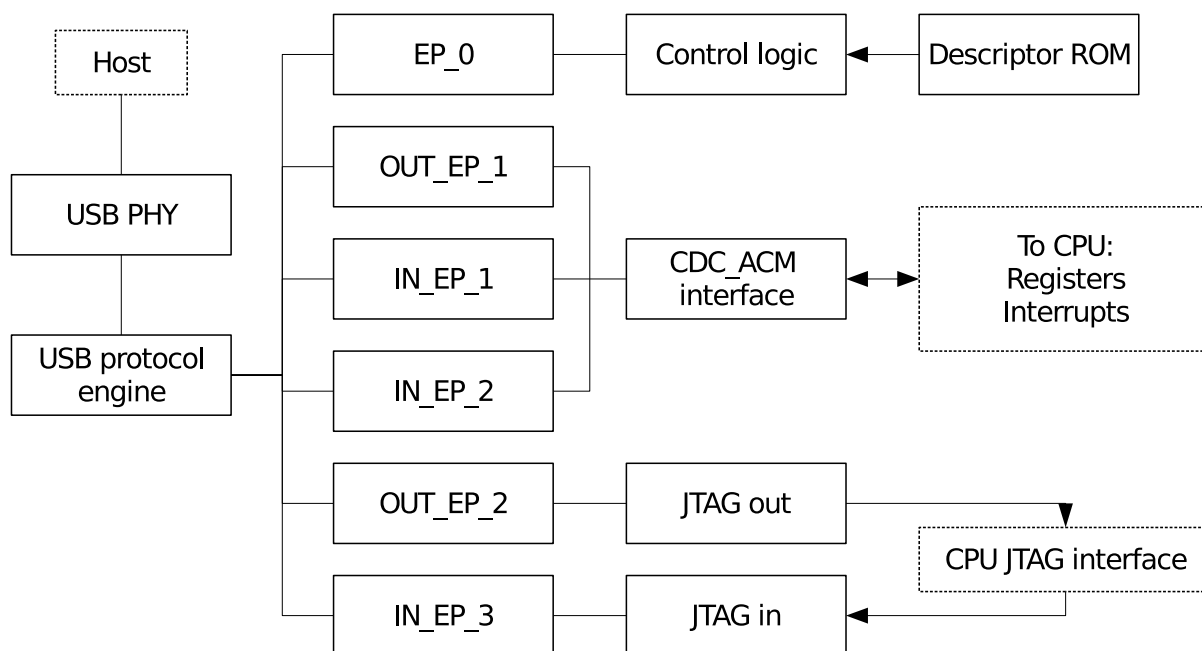
图 30-2. USB Serial/JTAG 框图
