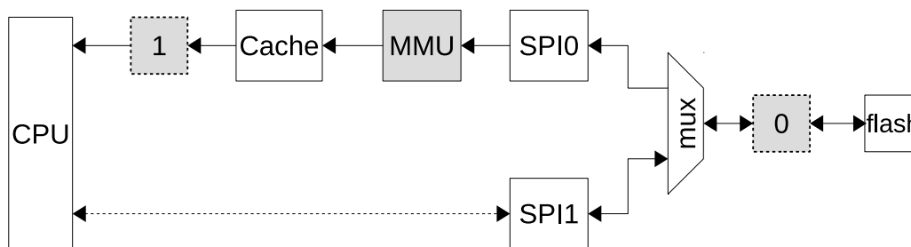
图 14-4. 外部存储器访问路径示意图
