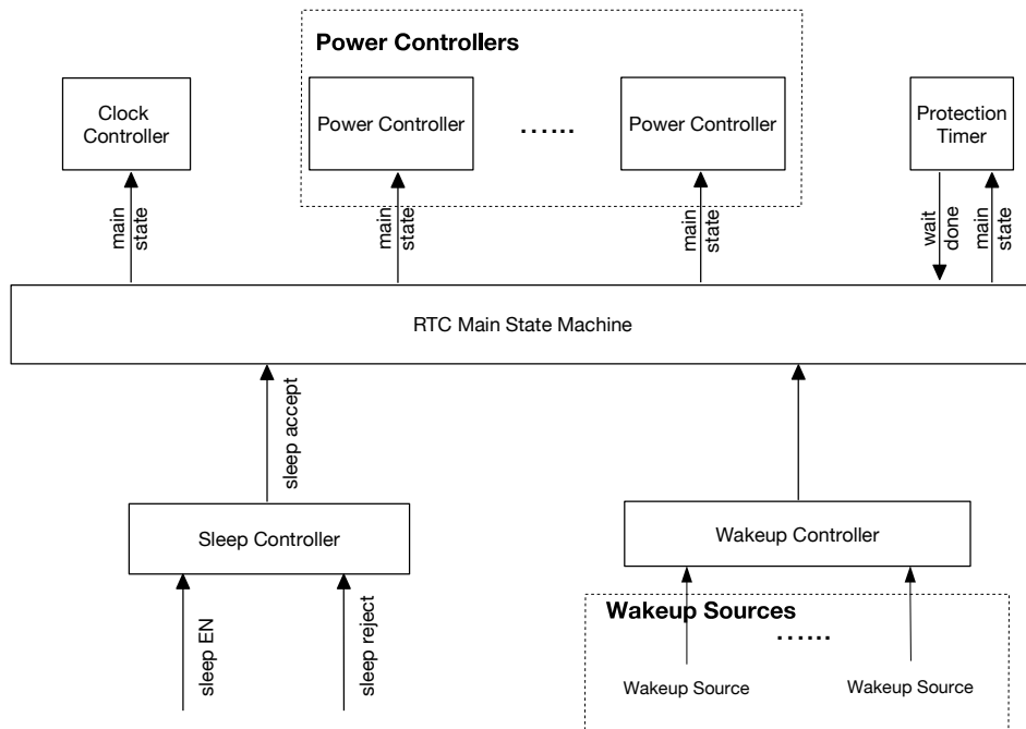
图 9-2. 电源管理单元的主要工作流程
