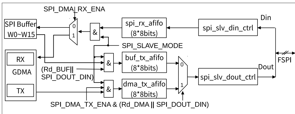
图 27-5. GP-SPI2 从机模式下的数据流控制
