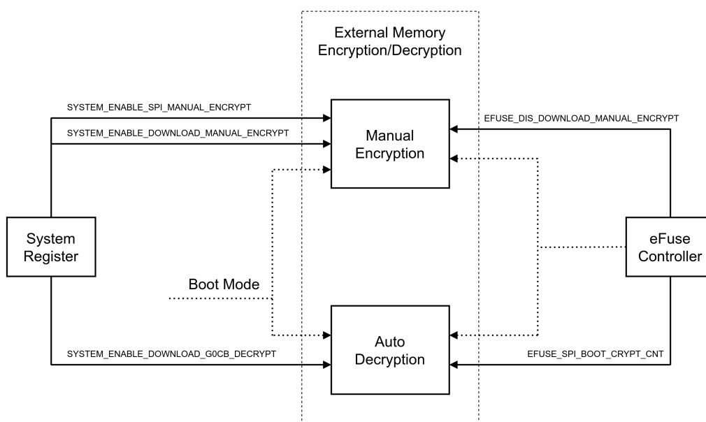
图 23-1. 片外存储器加解密结构
