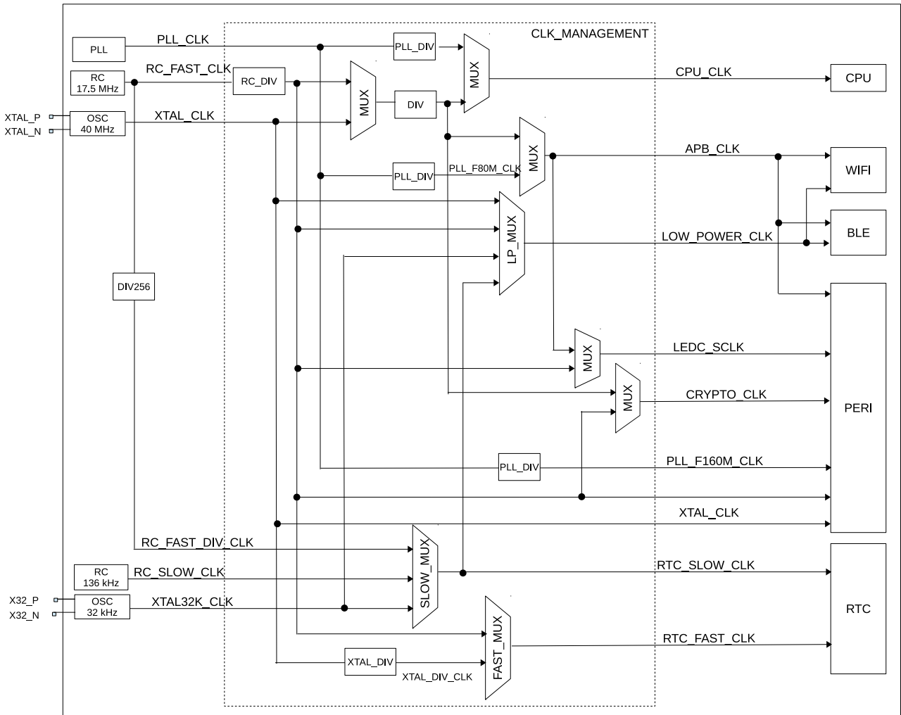
图 6-2. 系统时钟
