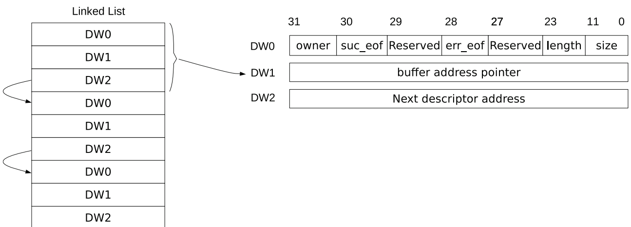
图 2-3. 链表结构图
