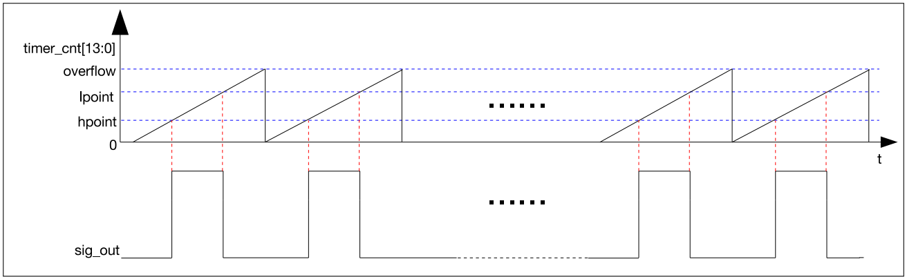
图 32-4. LED PWM 输出信号图
