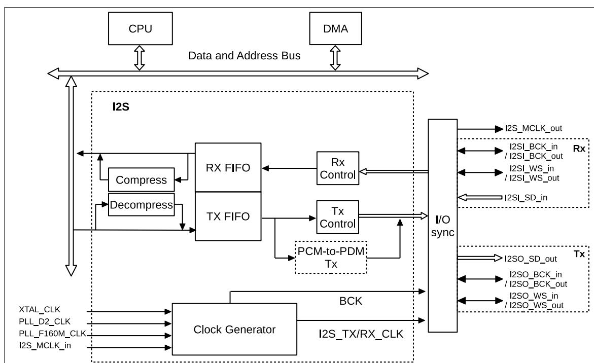
图 29-1. ESP32-C3 I2S 系统框图
