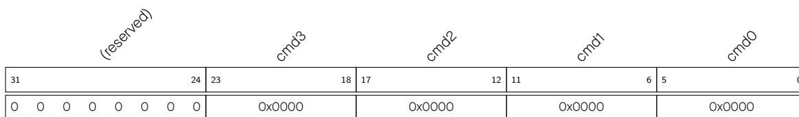
图 34-3. APB_SARADC_SAR_PATT_TAB1_REG 与样式 0 - 3
