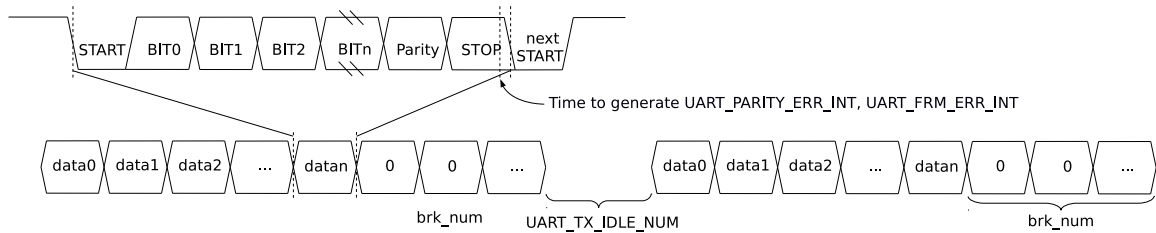
图 26-6. UART 数据帧结构
