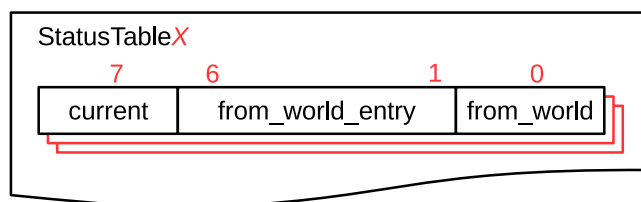
图 15-3. 世界切换记录表
