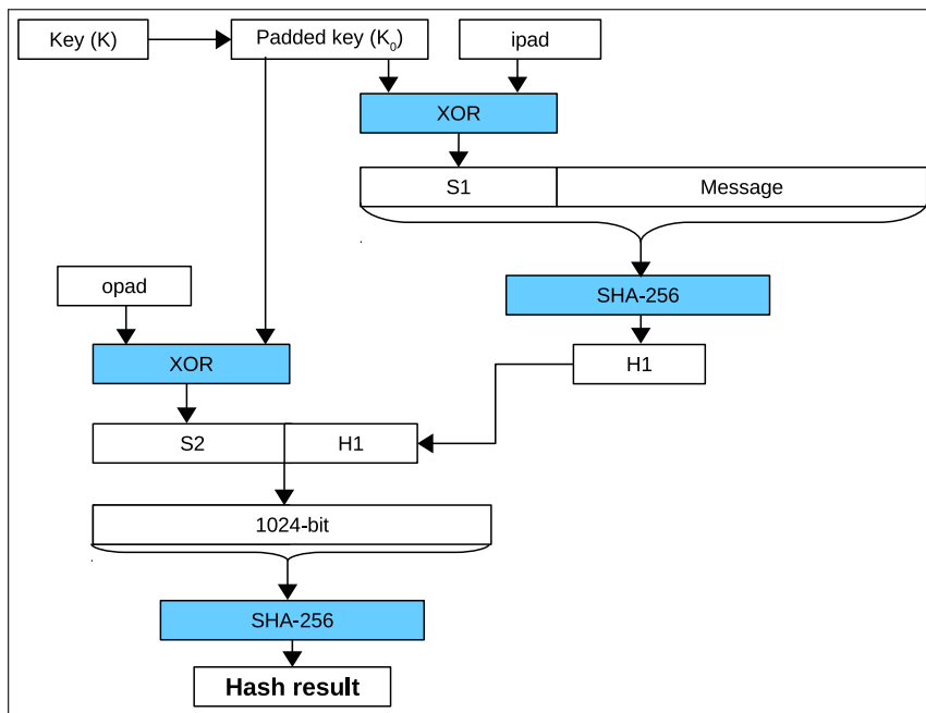
图 21-2. HMAC 结构示意图
