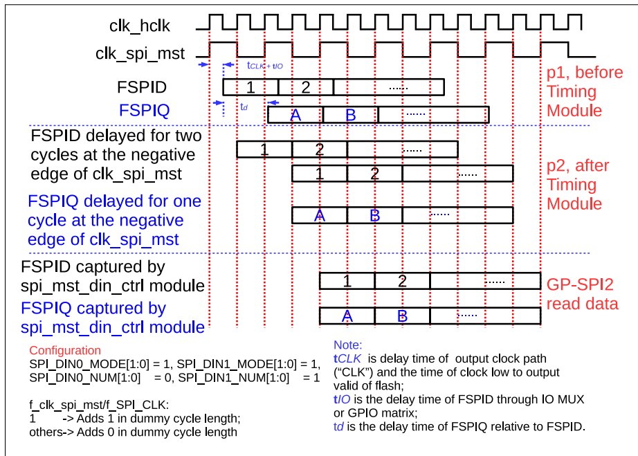
图 27-16. GP-SPI2 主机模式下时序补偿示例
