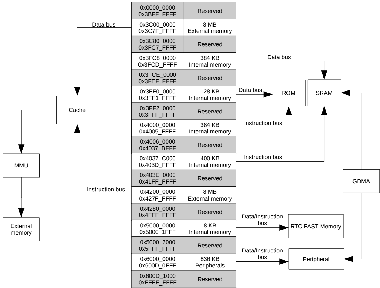
图 3-1. 系统结构与地址映射结构
